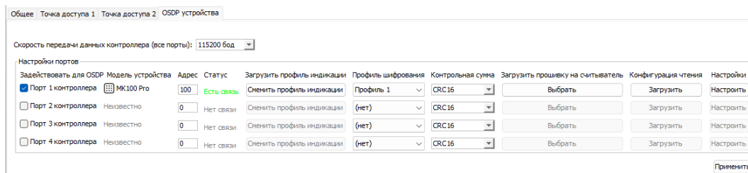
Проверка состояния связи по OSDP после применения профиля шифрования.
