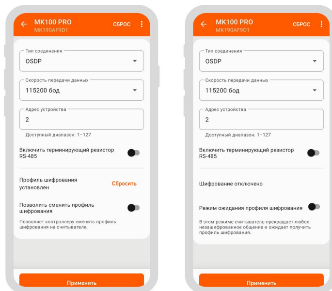
Процедура сброса профиля шифрования OSDP на считывателе.
