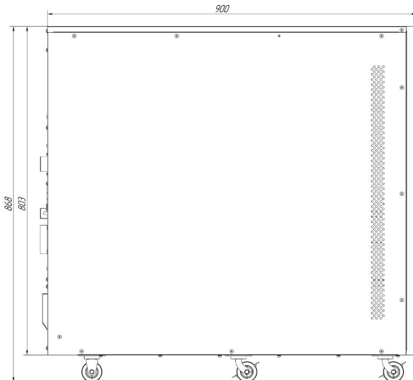
Вид сбоку
