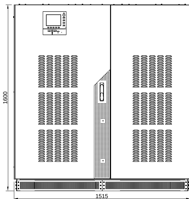
Вид спереди
