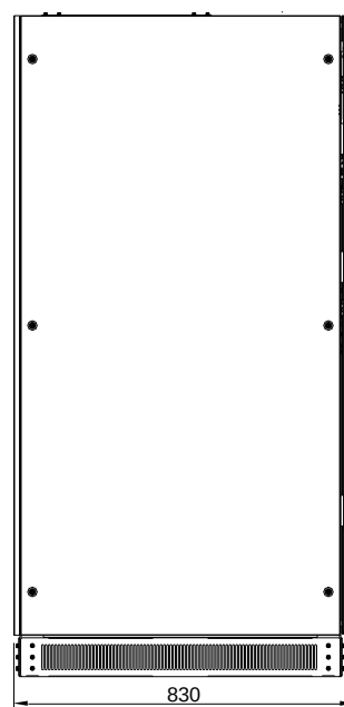
Вид сбоку
