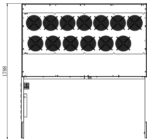
Вид сверху
