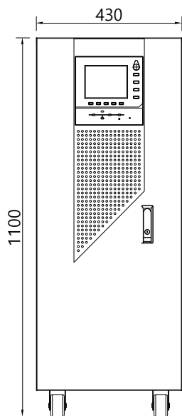
Вид спереди
