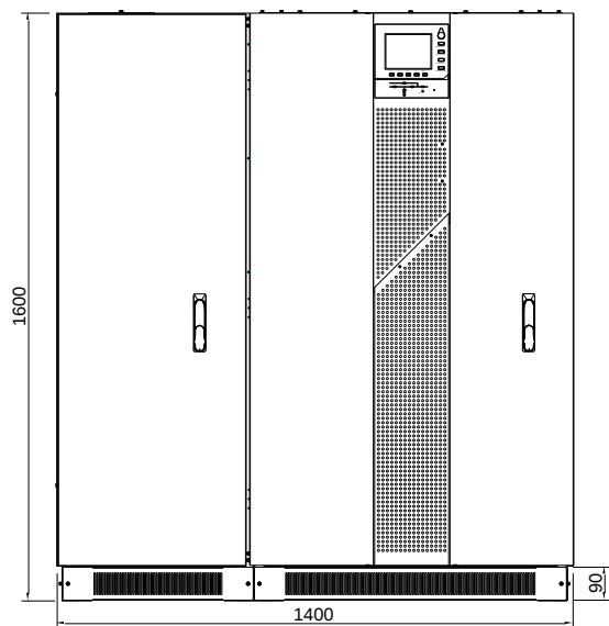
Вид спереди
