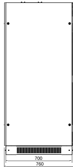
Вид сбоку
