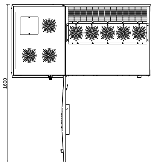
Вид сверху
