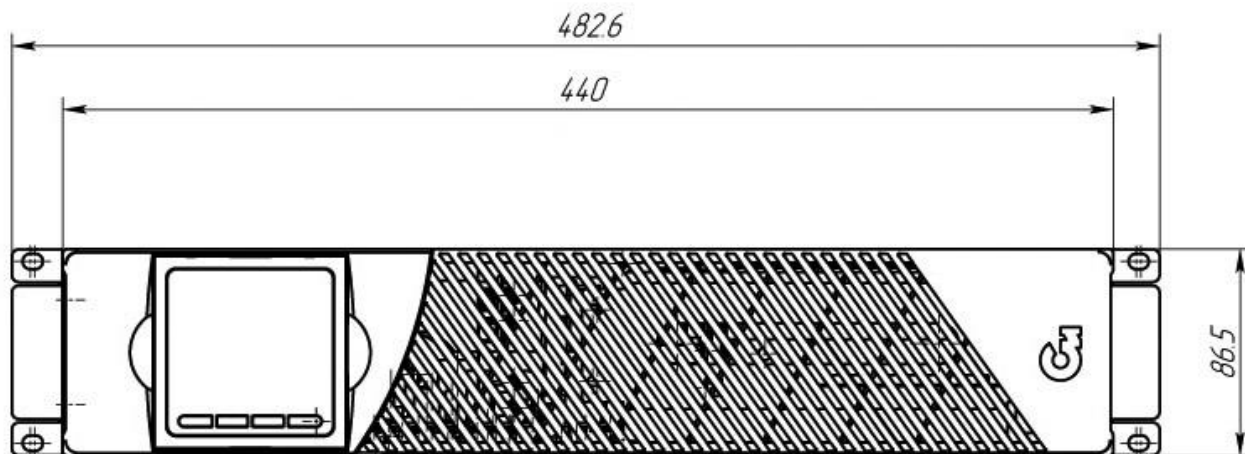
Габаритный чертеж ИБП СИПБ1,5КА.10-11
