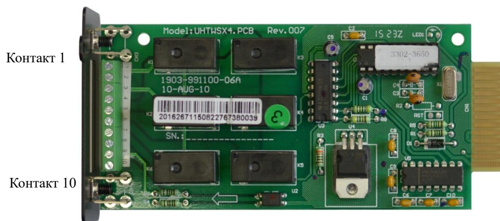
Внешний вид платы реле
