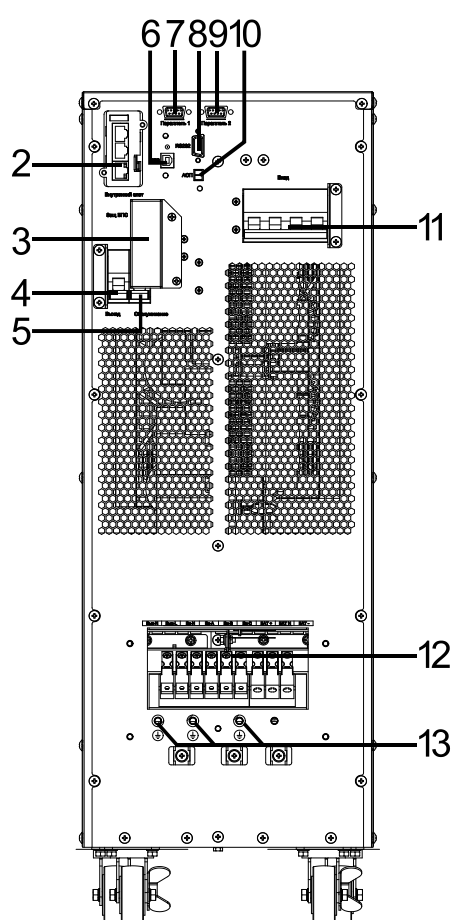
Задняя панель со снятой крышкой
