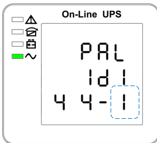
Настройки количества параллельно резервируемых устройств (Примечание: Область внутри пунктирной линии будет мигать)
