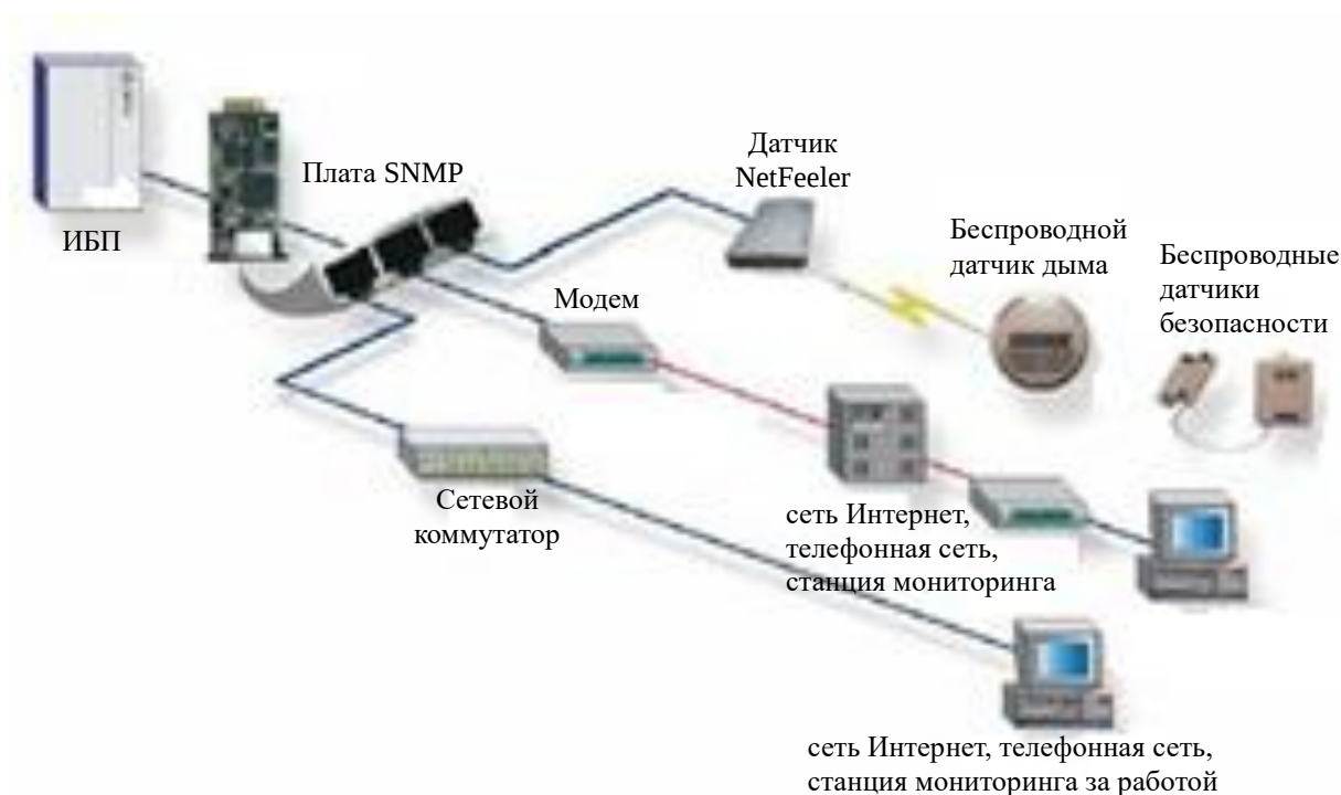
Стандартная топология сетевого управления ИБП
