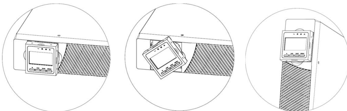
Рисунок 11 Поворот ЖК-дисплея ИБП при напольной установке
