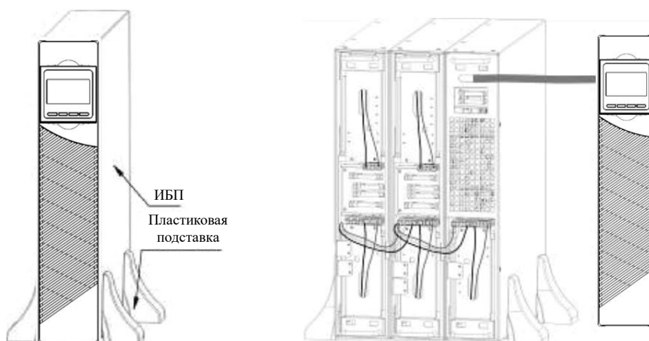
Рисунок 12 Напольная установка ИБП и батарейных блоков
