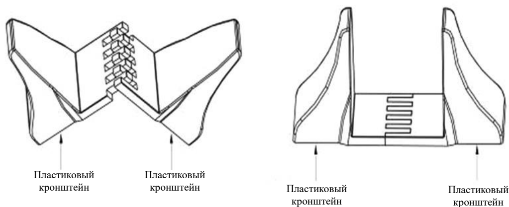
Рисунок 9 Сборка пластиковых подставок
