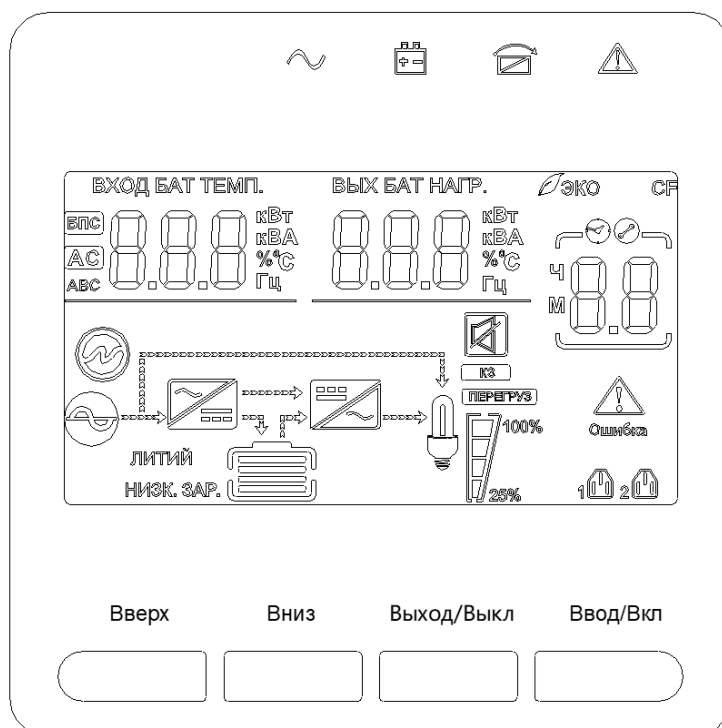
Внешний вид панели управления с ЖК-дисплеем
