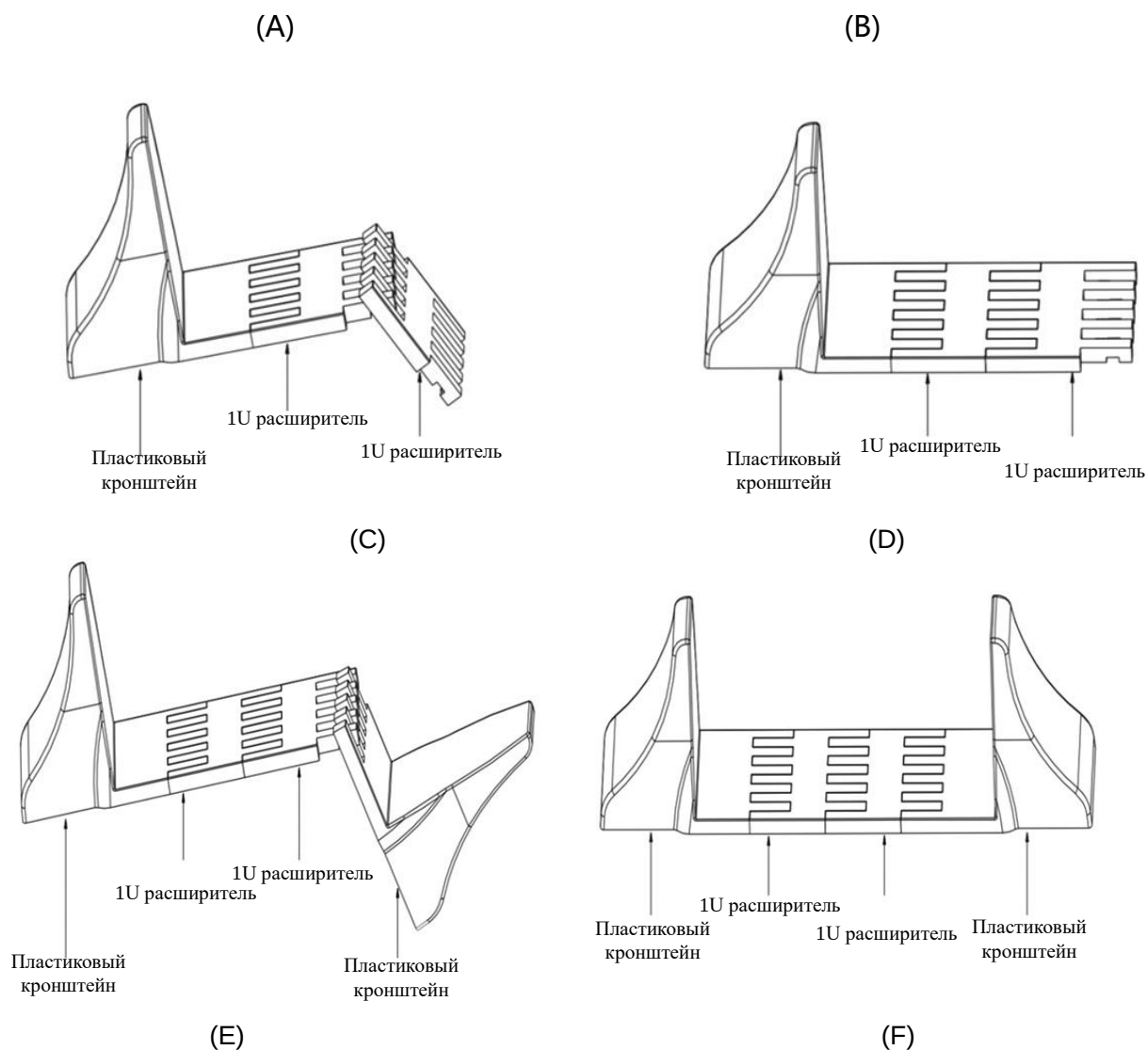
Рисунок 10 Расширение базы подставки
