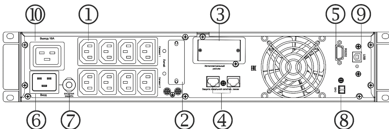
Рисунок 3. ИБП 3 кВА: вид сзади
