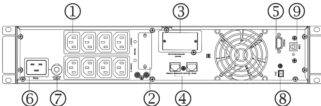
Рисунок 2. ИБП 2 кВА: вид сзади.
