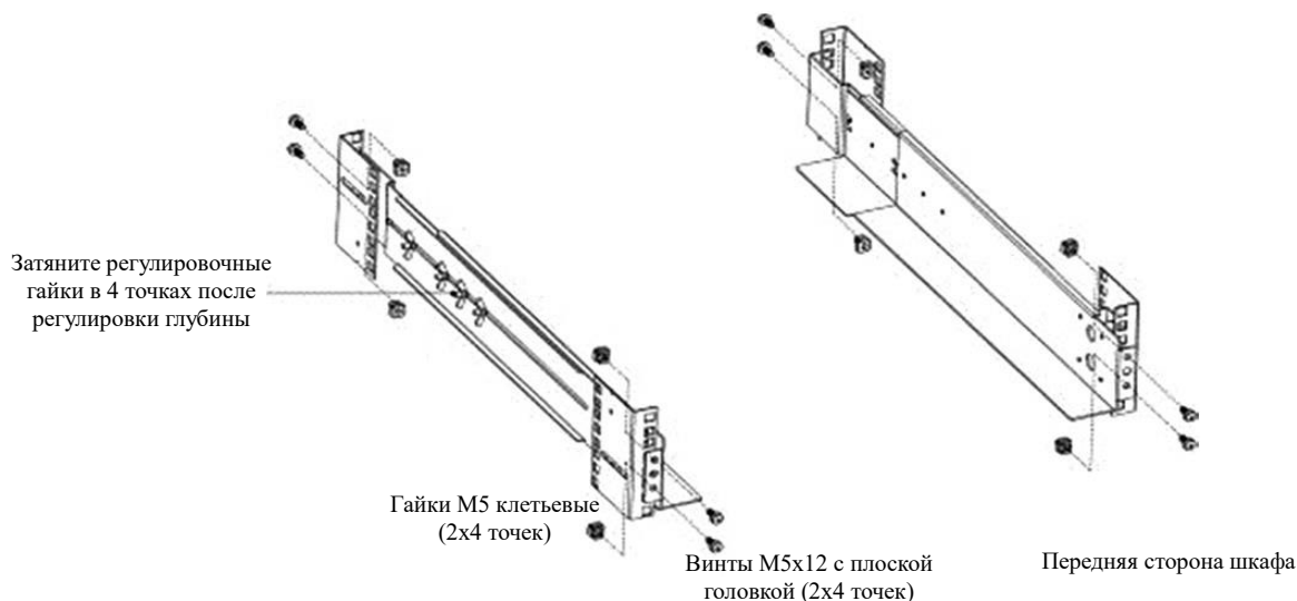
Рисунок 5. Крепление рельс
