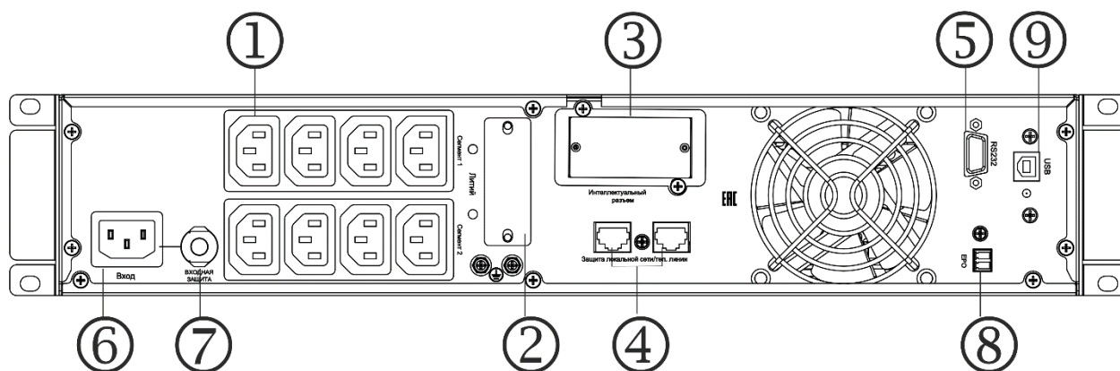
Рисунок 1. ИБП 1кВА: вид сзади.
