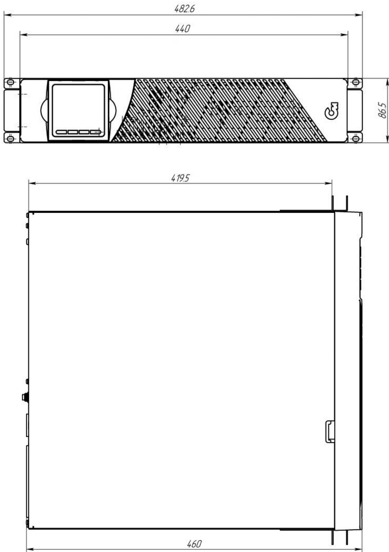
Габаритный чертеж ИБП СИПБ1КА.10-11
