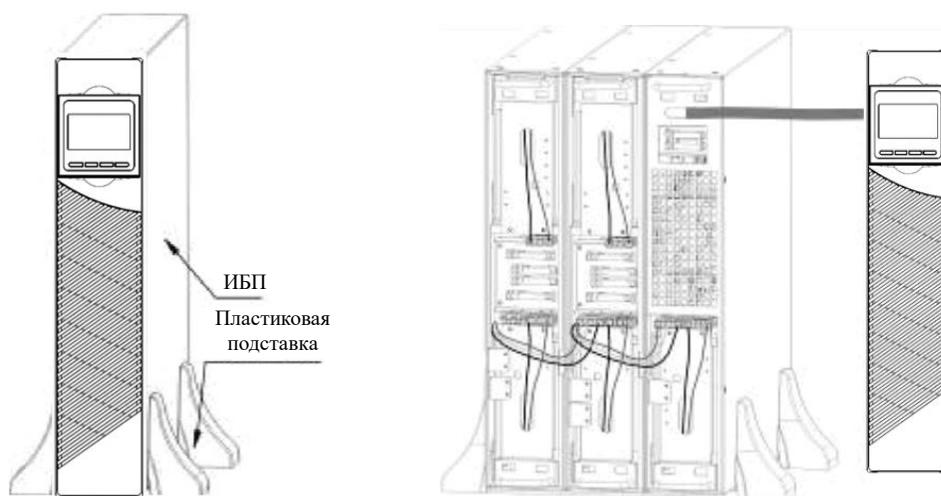
Рисунок 13 Напольная установка ИБП и батарейных блоков
