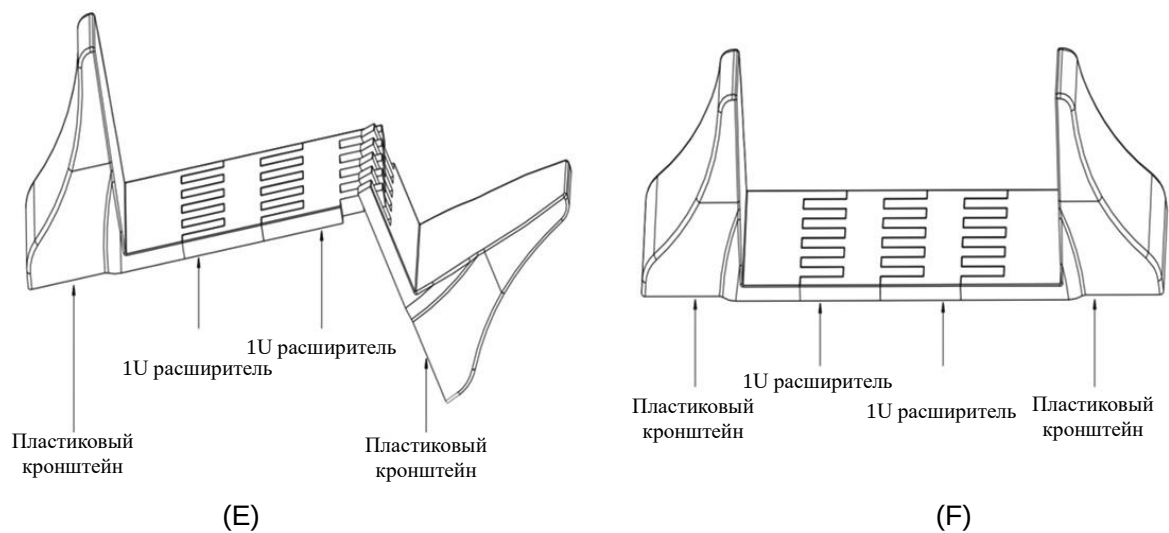
Рисунок 11 Расширение базы подставки
