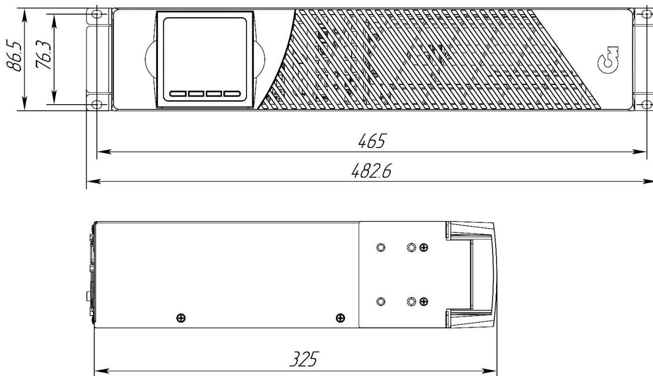
Габаритный чертеж ИБП СИПБ1КД.10-11
