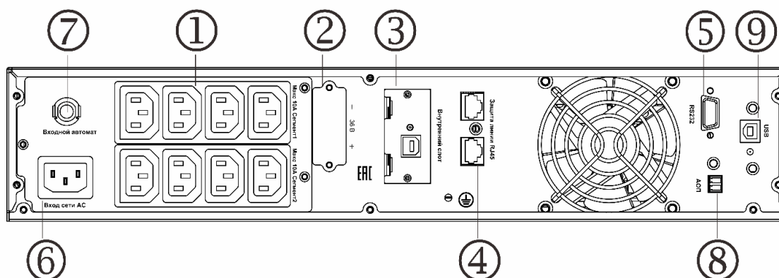
Задняя панель ИБП
