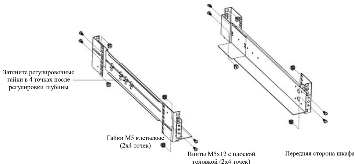
Рисунок 2 Крепление рельс
