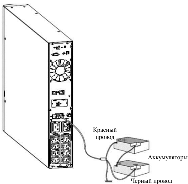
Рисунок 14 Подключение внешних батарей к ИБП с увеличенным временем работы
