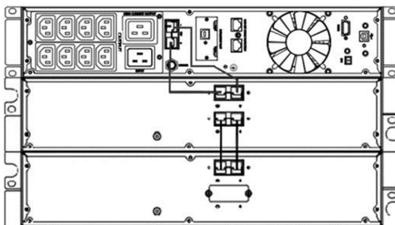
Рисунок 13 Подключение внешних батарейных блоков к ИБП через заднюю панель
