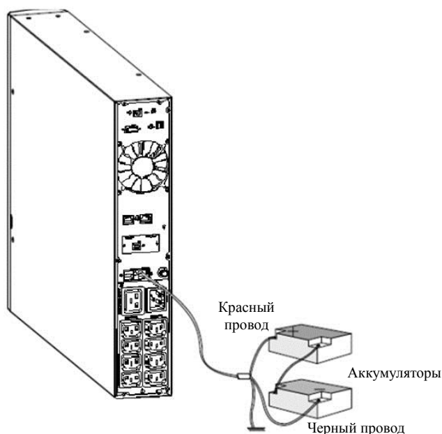
Рисунок 15 Подключение внешних батарей к ИБП с увеличенным временем работы
