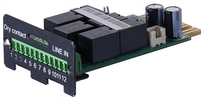
Внешний вид мини карты релейного интерфейса
