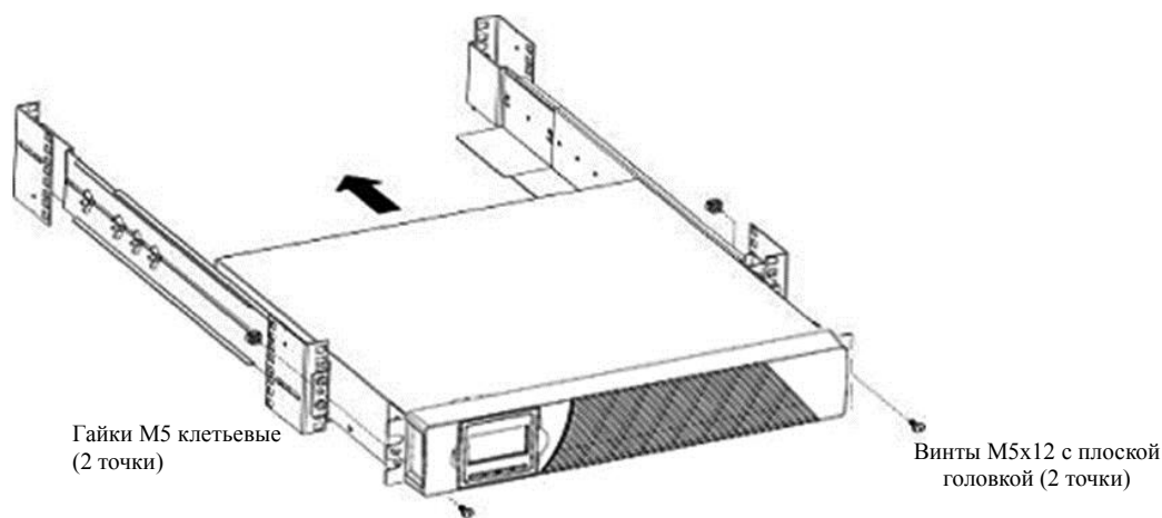
Рисунок 4 Крепление ИБП в шкафу спереди
