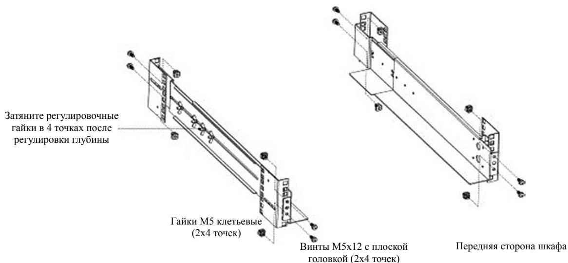
Рисунок 2 Крепление рельс
