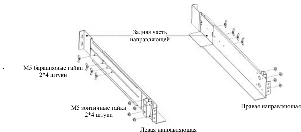
Рисунок 1 Сборка направляющих
