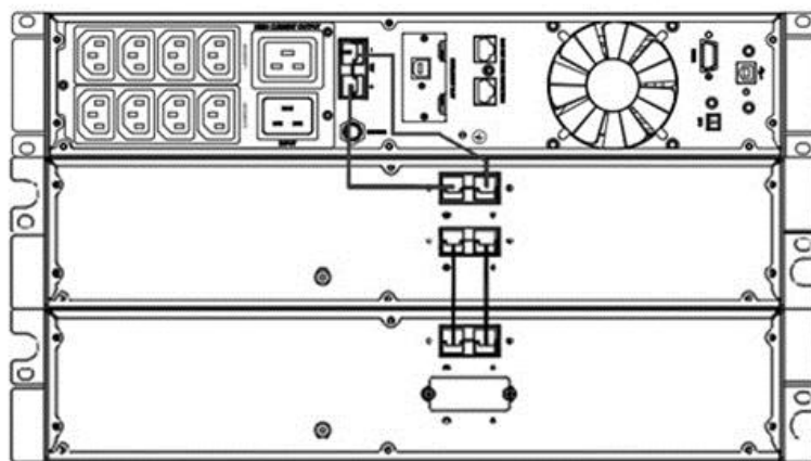
Рисунок 8 Подключение батарейного блока
