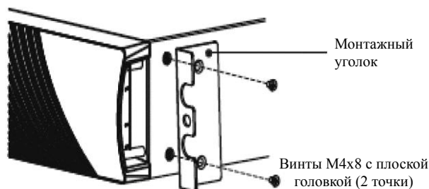
Рисунок 3 Установка монтажных кронштейнов
