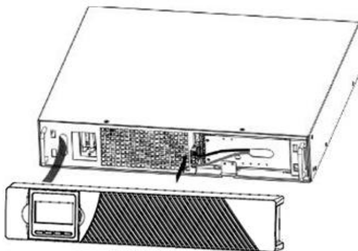
Рисунок 6 Подключение внутренних батарей ИБП
