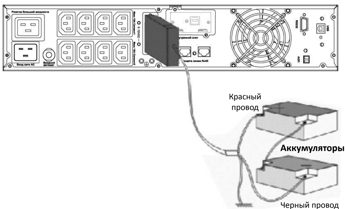
Рисунок 9 Подключение внешних аккумуляторных батарей
