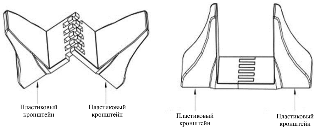
Рисунок 10 Сборка пластиковых подставок
