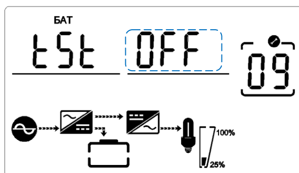
Тестирование аккумуляторов
