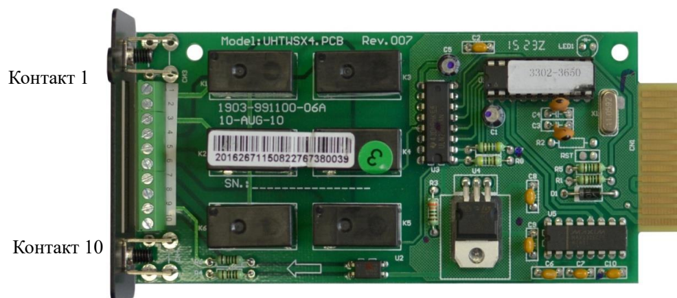
Внешний вид платы реле
