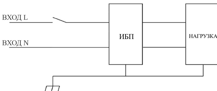
Схема соединения — «однофазная с заземлением»
