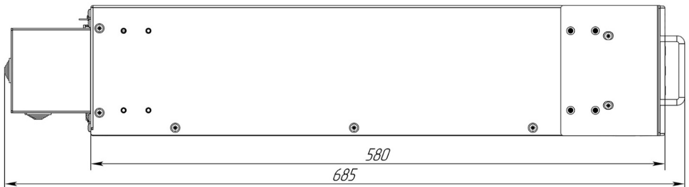
Вид сбоку
