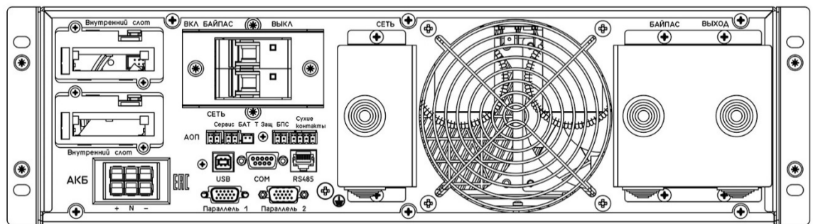
Вид сзади
