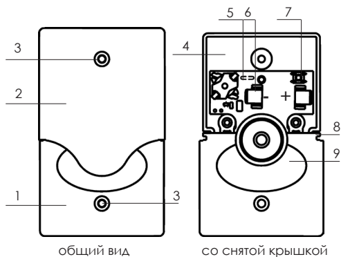
Рисунок 2 – Конструкция «Ri-S-1»
