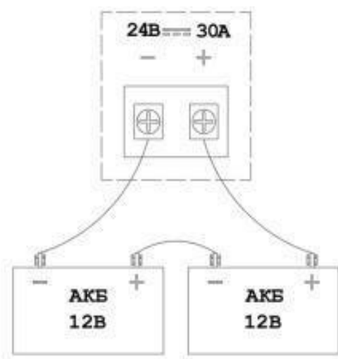
Рис. 3.1. Схема подключения АКБ к LPA-PRESTA-16
