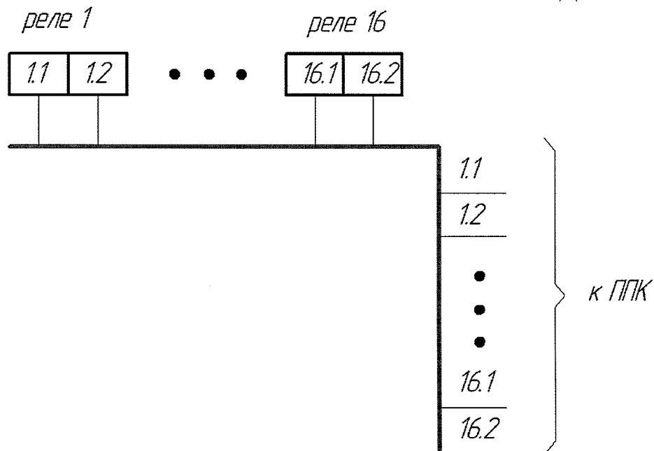
Рисунок 2.6 – Коммутация блока коммутации с ППК
