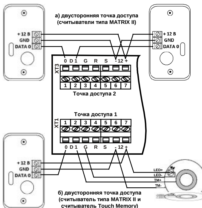
Рис. 8 Подключение считывателей при двусторонней ТД
