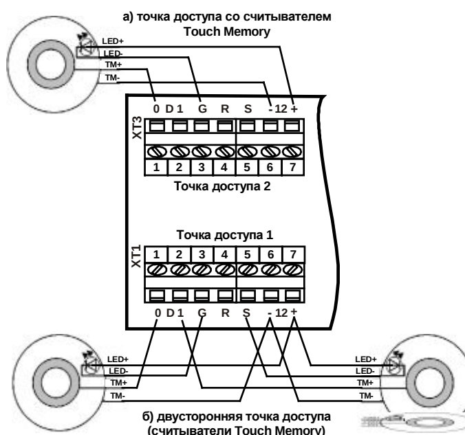
Рис. 9 Примеры подключения считывателей Touch Memory
