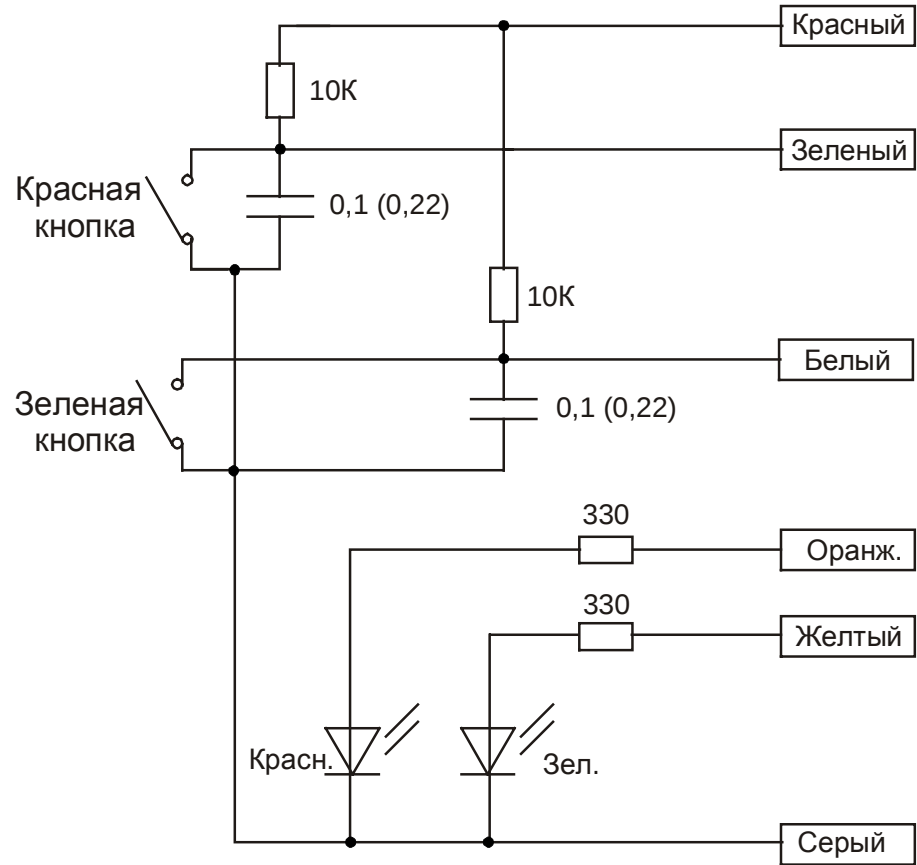
Рис. 8 Принципиальная схема подключения устройства постановки-снятия
