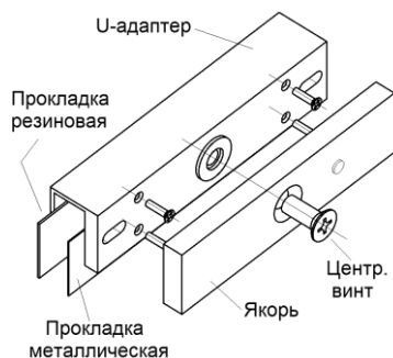
Рисунок 3 – Применение U-адаптера
