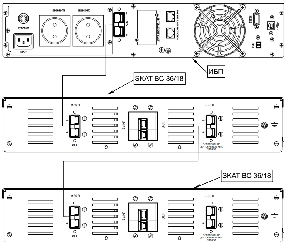
Рисунок 5 — Подключение ИБП и дополнительного батарейного блока
