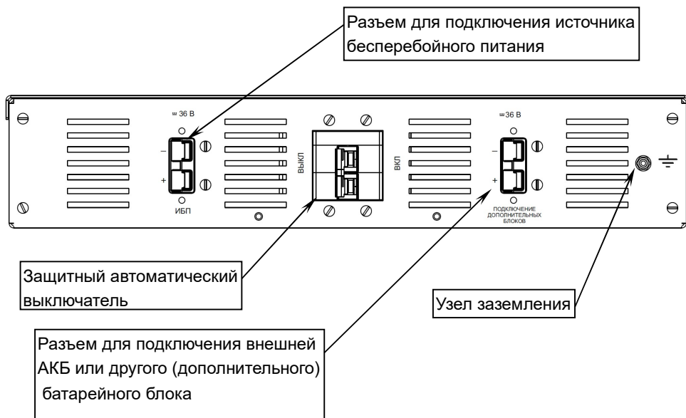
Рисунок 2 – Общий вид задней панели изделия со снятыми заглушками разъемов
