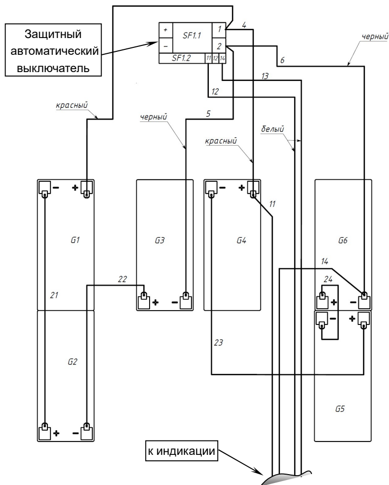
Рисунок 7 — Схема соединений аккумуляторных батарей
