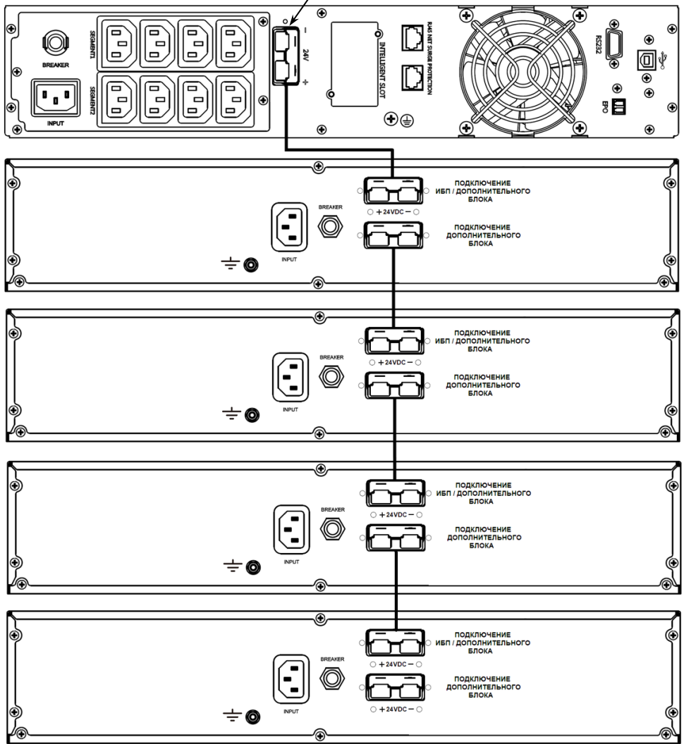
Рисунок 6 – Схема подключения нескольких ББ к ИБП (Продолжение на стр. 11)
