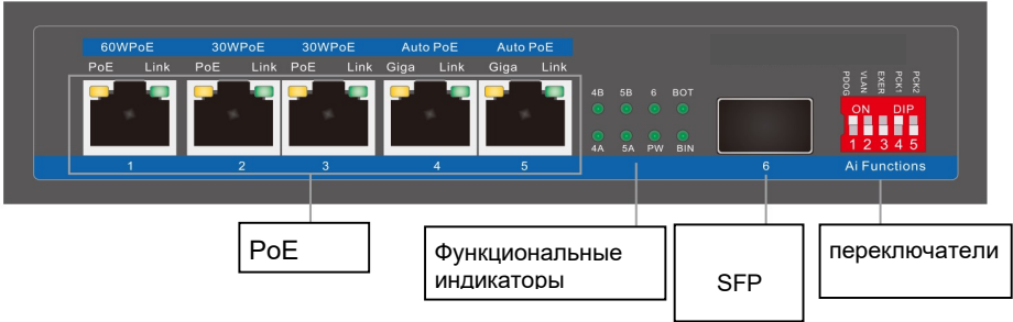
Рисунок 1 – Передняя панель изделия
