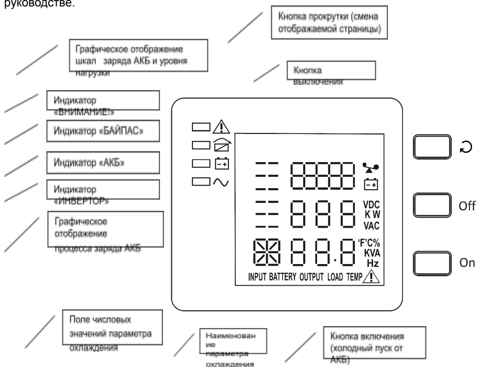
Рисунок 3 - ЖК—дисплей
