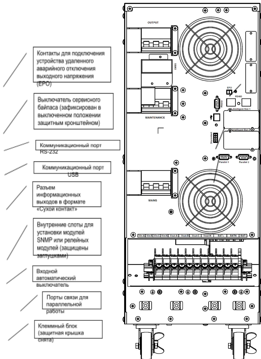
Рисунок 2 — Общий вид задней панели изделия со снятой крышкой клеммного блока
