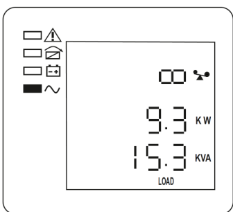
Рисунок 17 — ЖК-дисплей, общая мощность нагрузки
