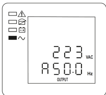
Рисунок 11 — ЖК-дисплей, Фаза А, выходное напряжение и частота
