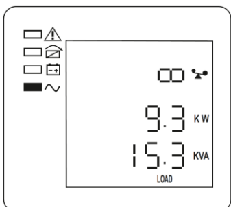
Рисунок 17 — ЖК-дисплей, общая величина нагрузки
