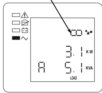
Рисунок 14 — ЖК-дисплей, Фаза А, мощность нагрузки
