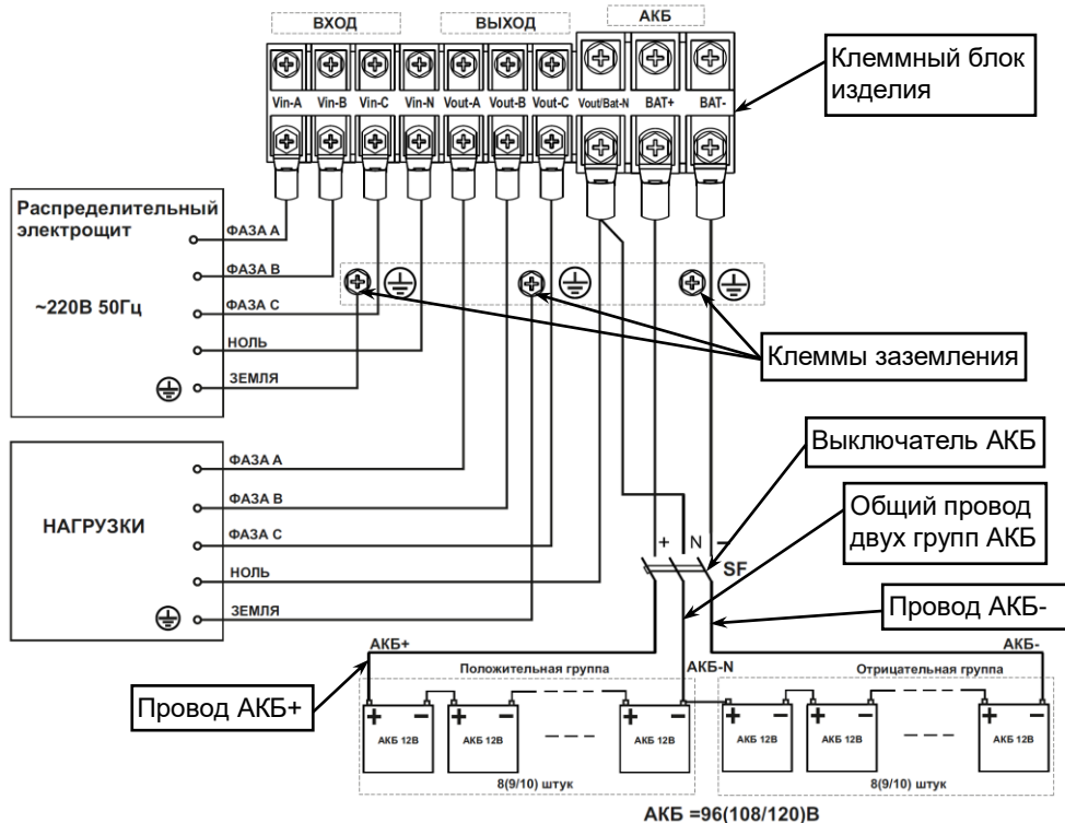
Рисунок 23 — Схема подключения изделия и монтажа аккумуляторной батареи.
