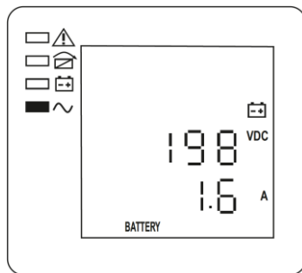
Рисунок 8 — ЖК-дисплей, положительная группа АКБ, напряжение и ток
