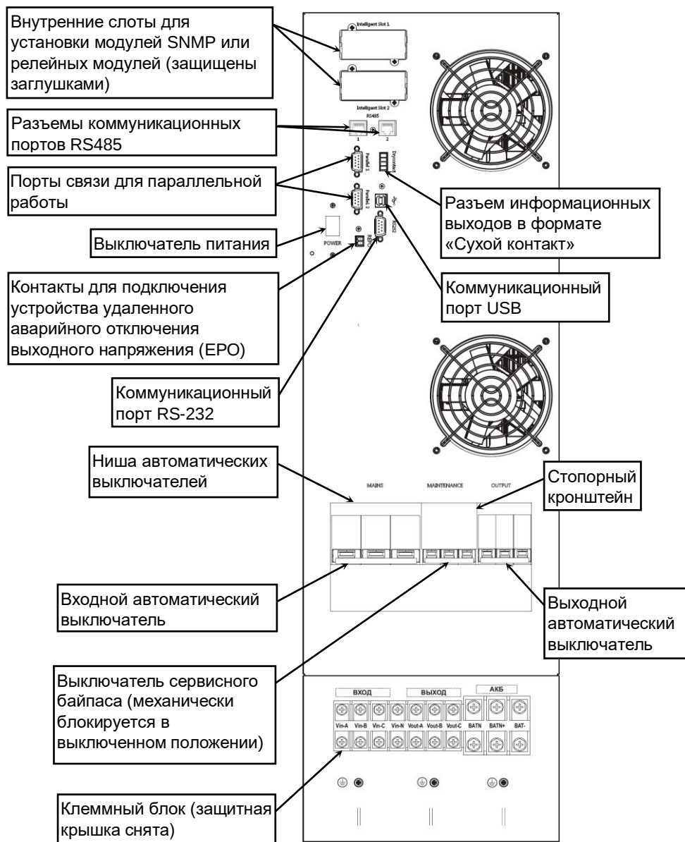
Рисунок 2 — Общий вид задней панели изделия со снятой крышкой клеммного блока
