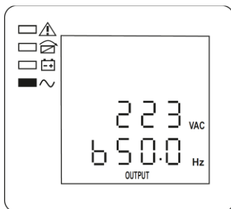
Рисунок 12 — ЖК-дисплей, Фаза В, выходное напряжение и частота
