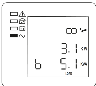
Рисунок 15 — ЖК-дисплей, Фаза В, величина нагрузки
