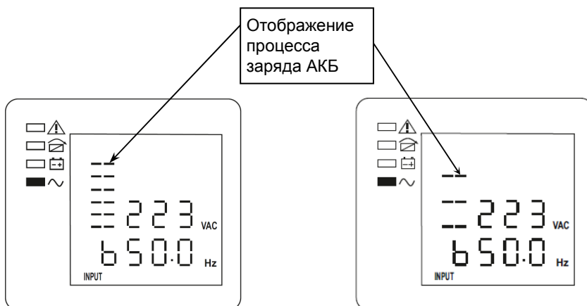
Рисунок 21 — ЖК-дисплей, форсированный (ускоренный) заряд АКБ
