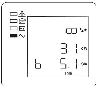
Рисунок 15 — ЖК-дисплей, Фаза В, мощность нагрузки
