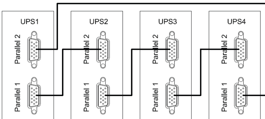
Рисунок 24 — Схема подключения изделий в систему параллельного резервирования.
