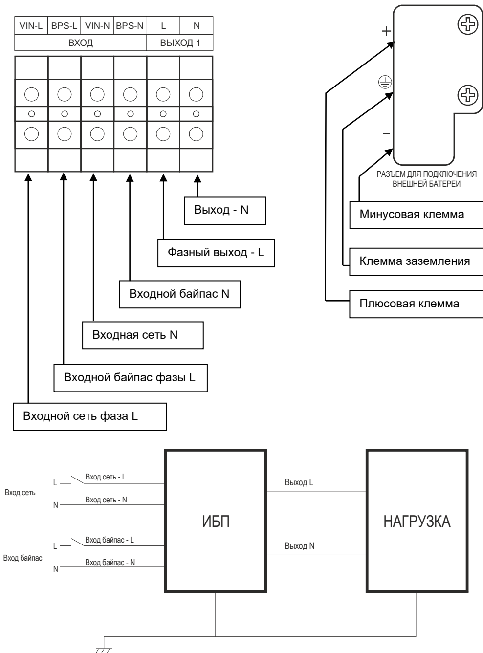
Рисунок 7 – Схема с раздельным вводом байпас
