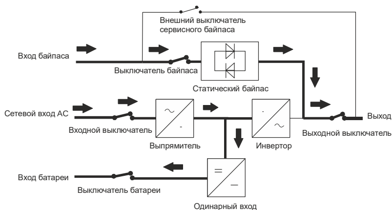
Рисунок 23 – Режим работы ECO с отдельным вводом байпас
