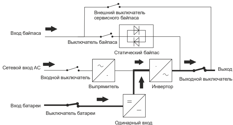
Рисунок 19 – Режим работы «РЕЗЕРВ» с отдельным вводом байпас
