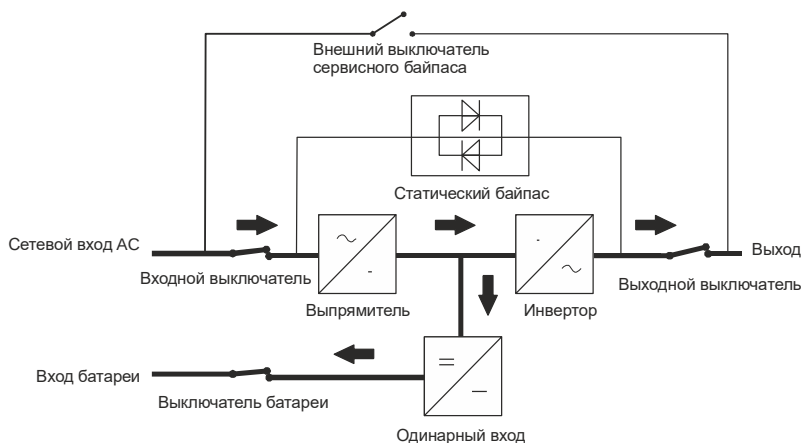
Рисунок 17 – Режим работы «ОСНОВНОЙ» с отдельным вводом байпас
