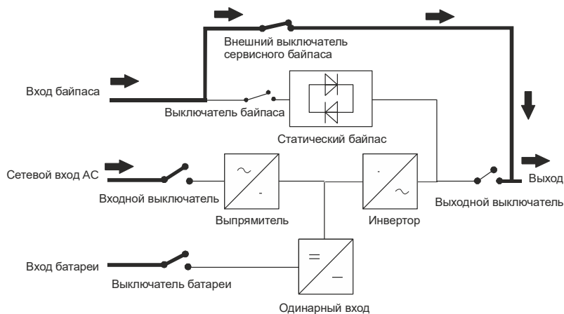
Рисунок 25 – Режим работы ручной байпас с отдельным вводом байпаса
