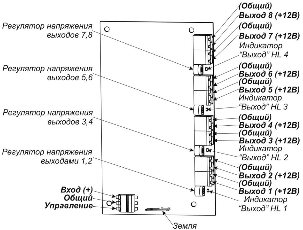
Расположение элементов коммутации, управления и индикации на плате преобразователя PN-V.8
