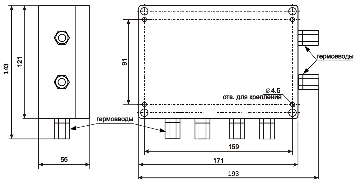
Рис. 3 Габаритные и присоединительные размеры СКАУ исп.2 IP65
