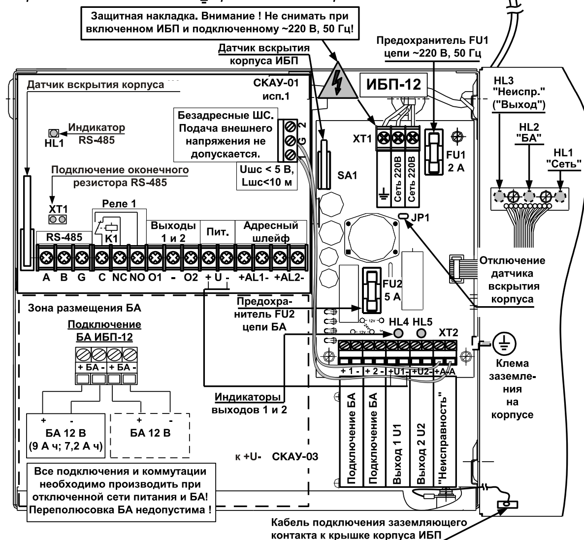
Рис. 4 Внешний вид СКАУ исп. 1
