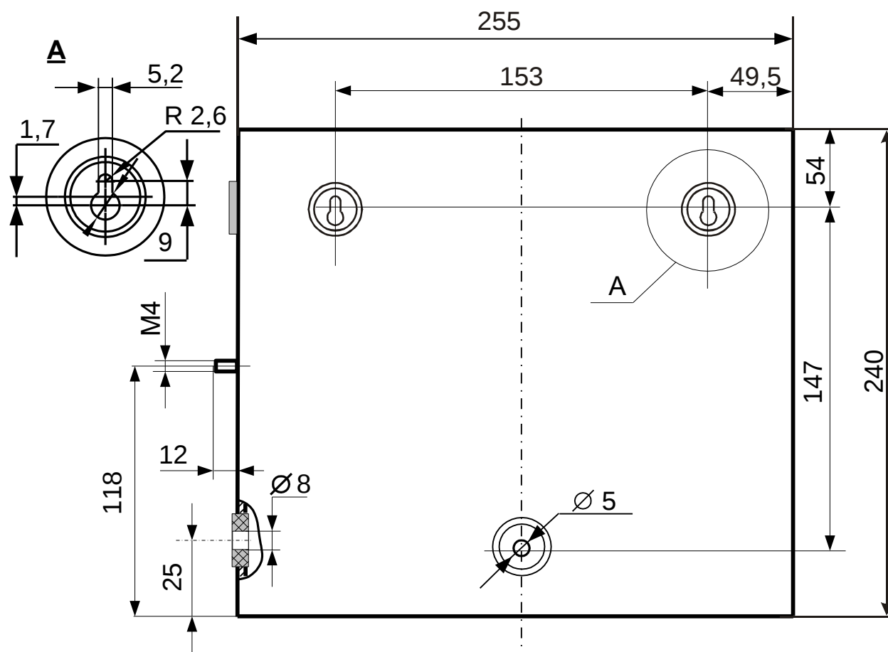
Рис. 5 Габаритные и присоединительные размеры СКАУ исп. 1
