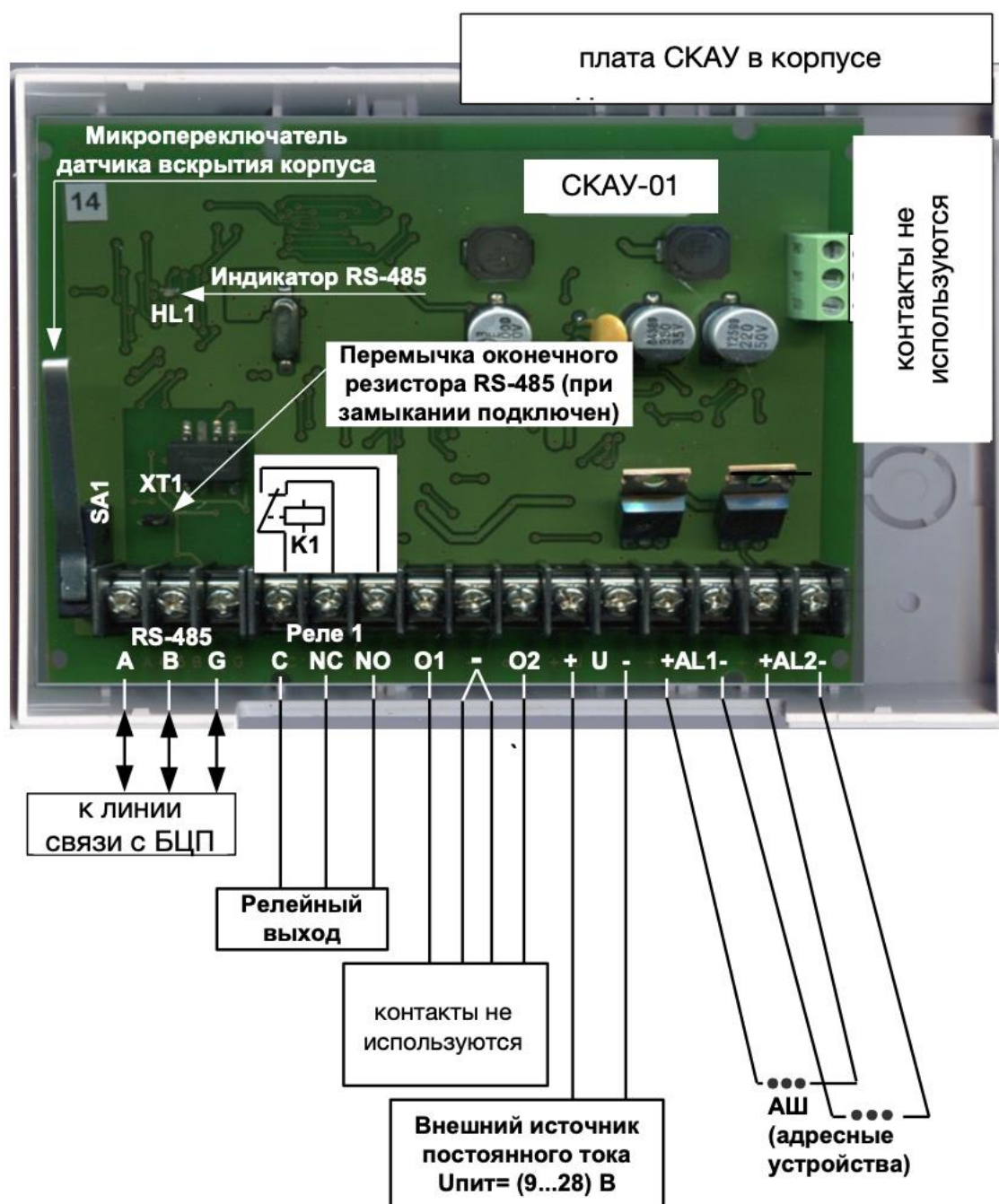
Рис. 1 Внешний вид СКАУ исп.2 IP20. Клеммы подключения.
