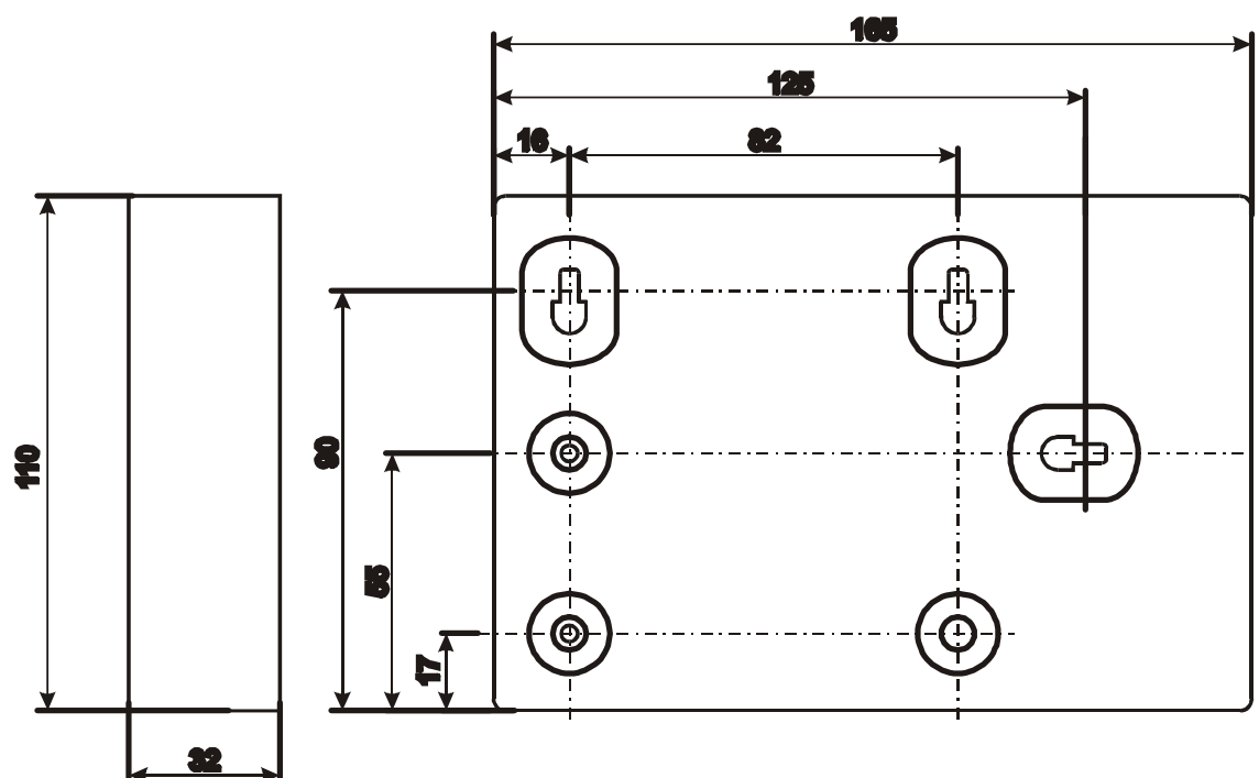
Рис. 2 Габаритные и присоединительные размеры СКАУ исп.2 IP20
