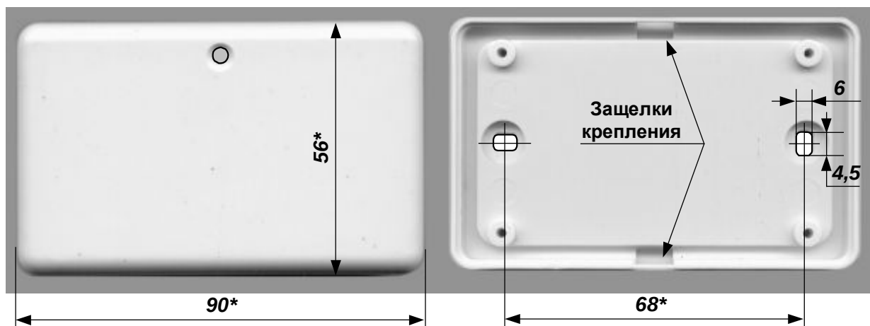
Рис. 3 Габаритные и присоединительные размеры корпуса SKAU-01-M1
