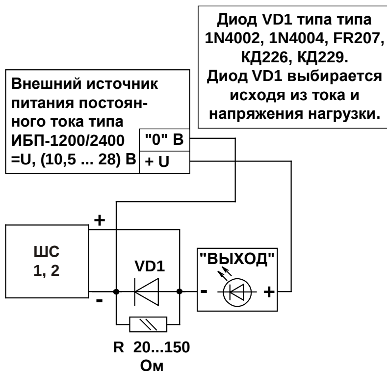
Рис. 4 Подключение светового оповещателя
