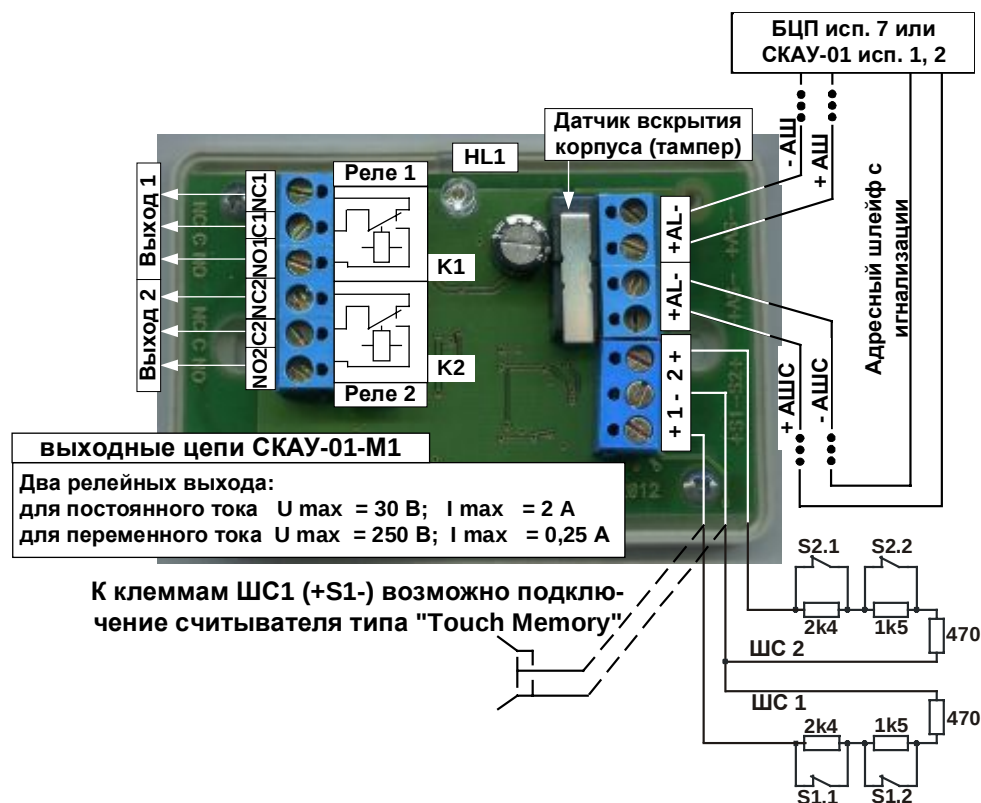
Рис. 2 Подключение СКАУ-01-M1
