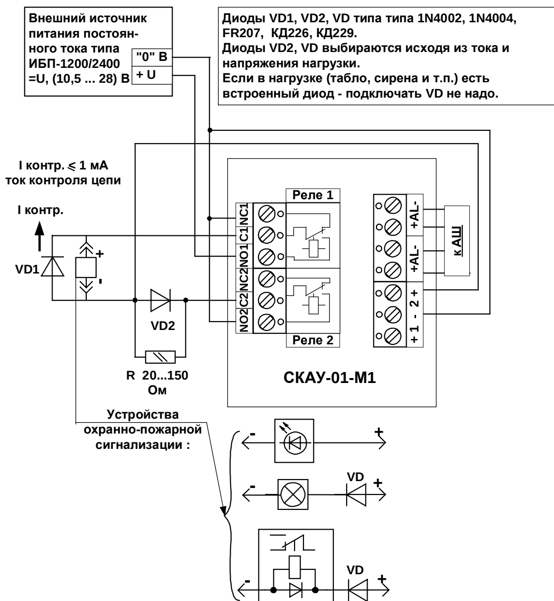
Рис. 5 Подключение исполнительных устройств к релейным выходам с контролем цепи управления
