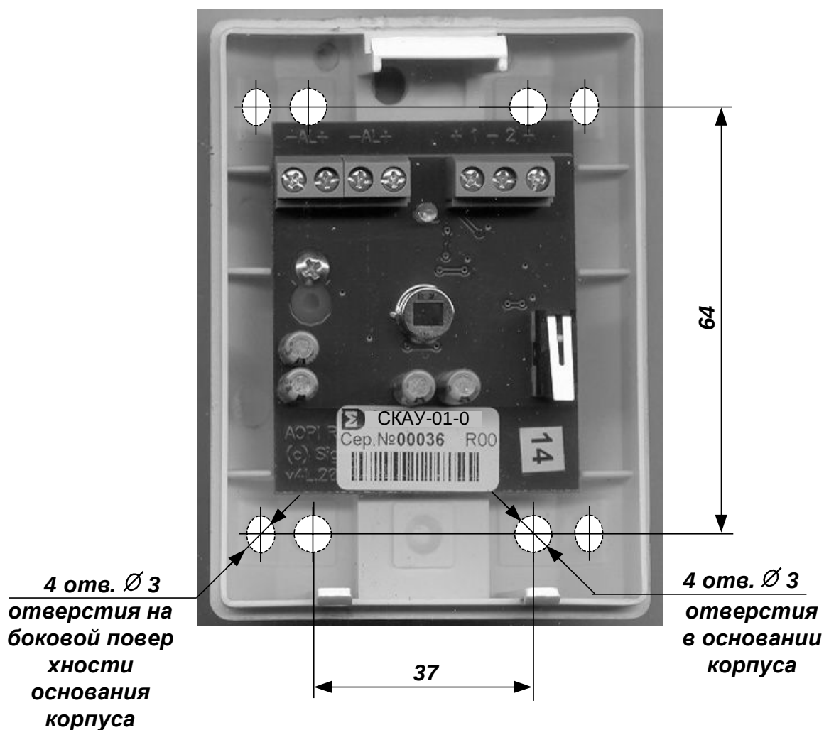
Рис. 4 Присоединительные размеры корпуса устройства
