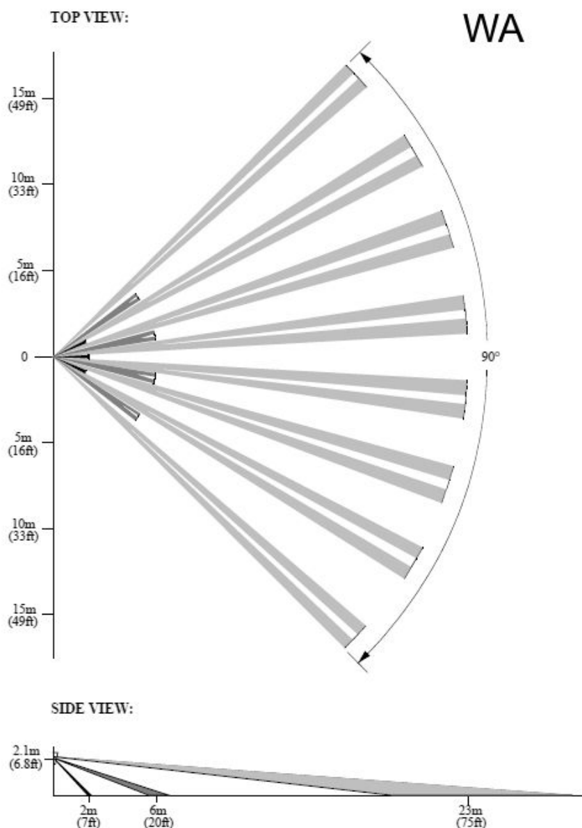
Рис. 5 Диаграмма зоны обнаружения при использовании линзы WA (вариант «О»)
