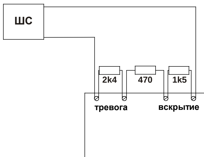
Рис. 7 Пример подключения в шлейф извещателя с отдельными клеммами датчика вскрытия и сигнала тревоги.
