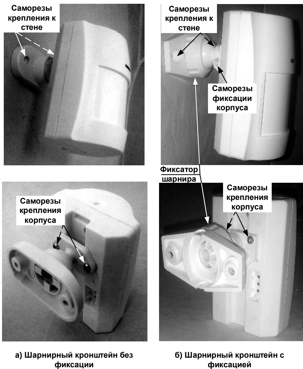
Рис. 9 Шарнирные кронштейны крепления: а) без фиксации; б) с фиксацией.
