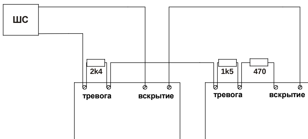
Рис. 8 Пример подключения в шлейф двух извещателей с отдельными клеммами датчика вскрытия и сигнала тревоги.
