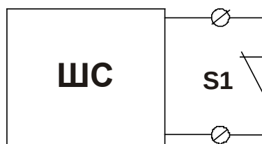
Рис. Схема 5 Подключение НЗ контактов без контроля целостности линии связи.
