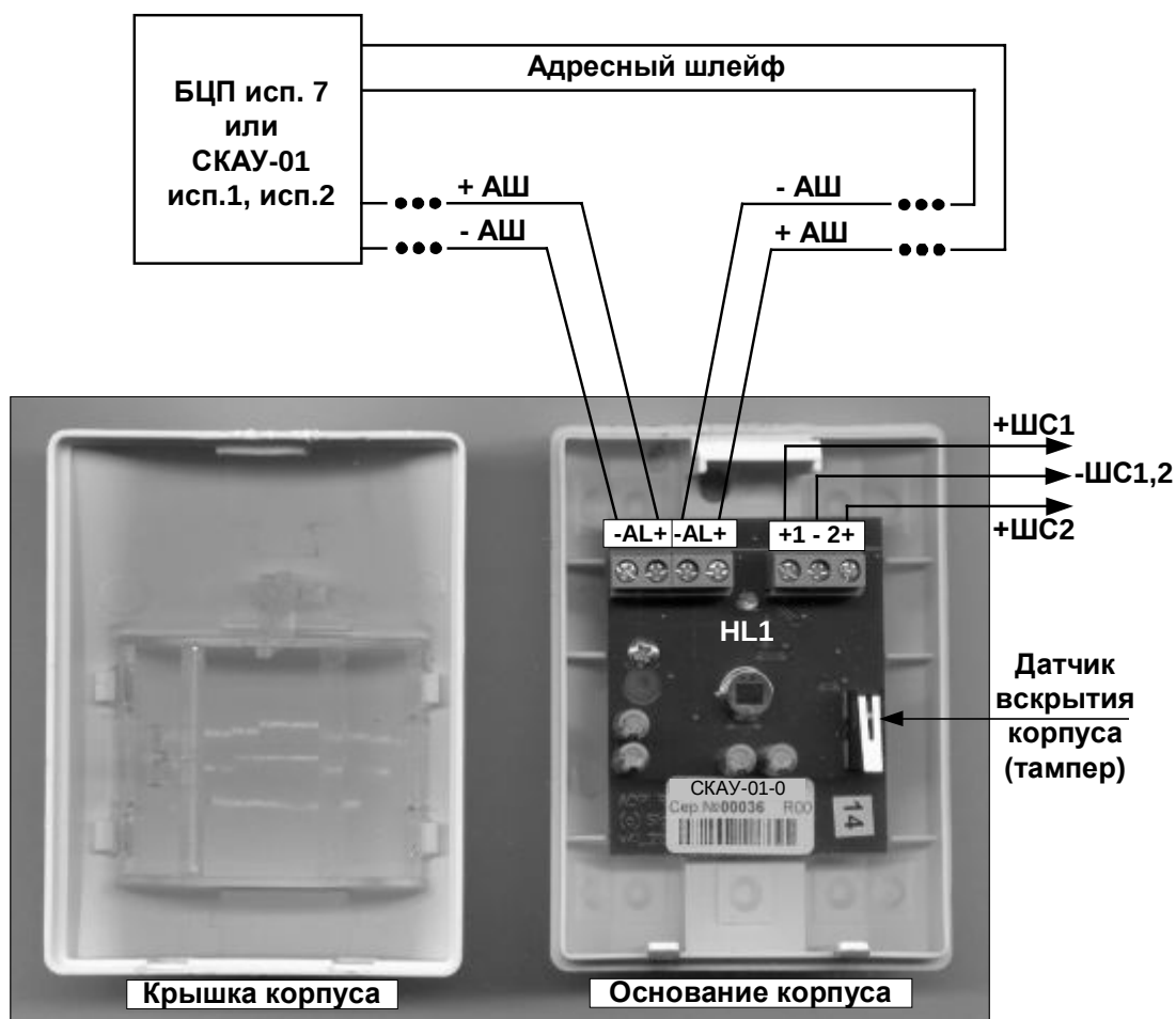
Рис. 3 Конструкция, подключение устройства
