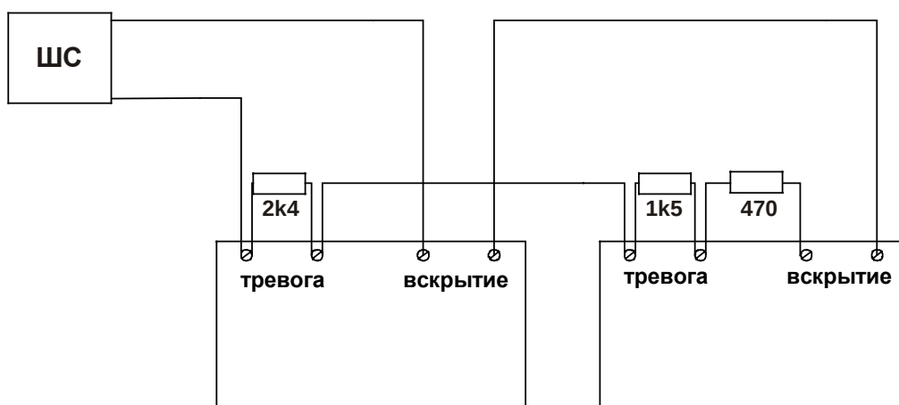
Рис. 11 Пример подключения в шлейф двух извещателей с отдельными клеммами датчика вскрытия и сигнала тревоги.
