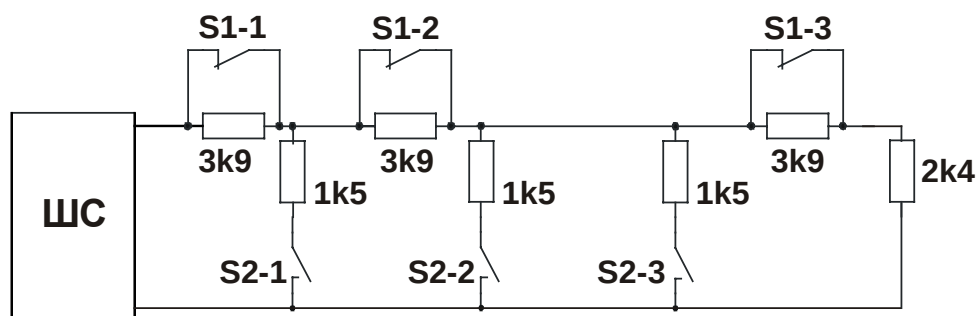
Рис. Схема 7. Параллельно-последовательное подключение НЗ и НР извещателей
