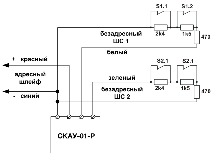
Рис. 6 Пример подключения 4-х извещателей с НЗ контактами.
