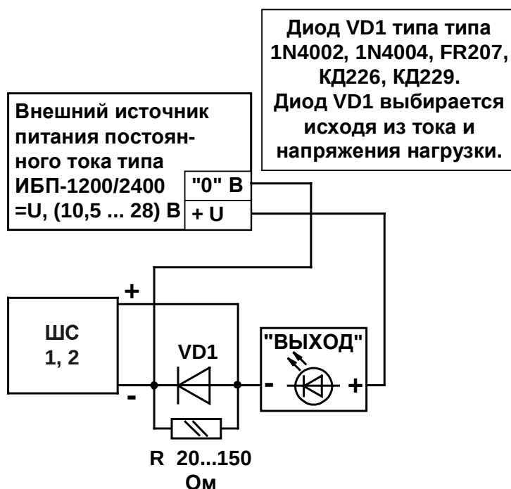
Рис. 9 Подключение светового оповещателя
