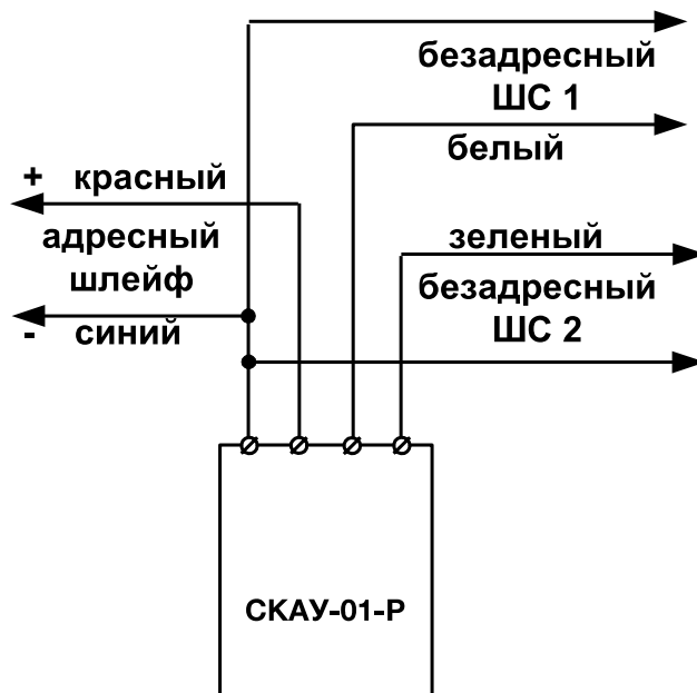
Рис. 5 Подключение двух шлейфов.
