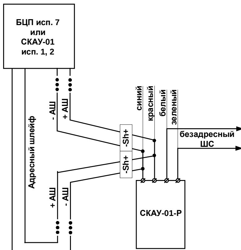
Рис. 3 Подключение устройства с одним ШС
