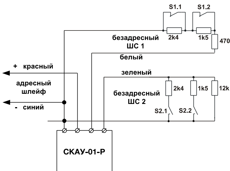
Рис. 8 Пример подключения 2-х извещателей с НЗ контактами и 2-х извещателей с НР контактами.
