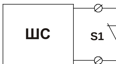
Рис. Схема 8 Подключение извещателя (датчика) с НЗ контактами без контроля целостности линии связи.
