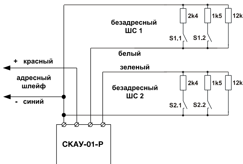
Рис. 7 Пример подключения 4-х извещателей с НР контактами.
