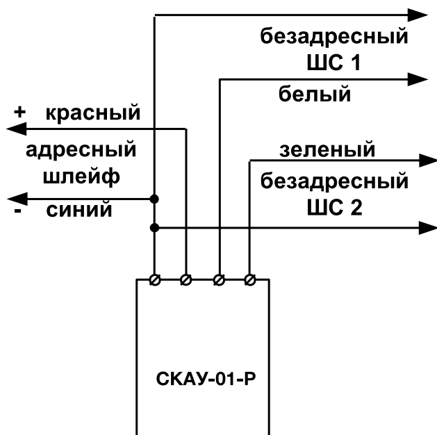
Рис. 4 Подключение устройства с двумя ШС
