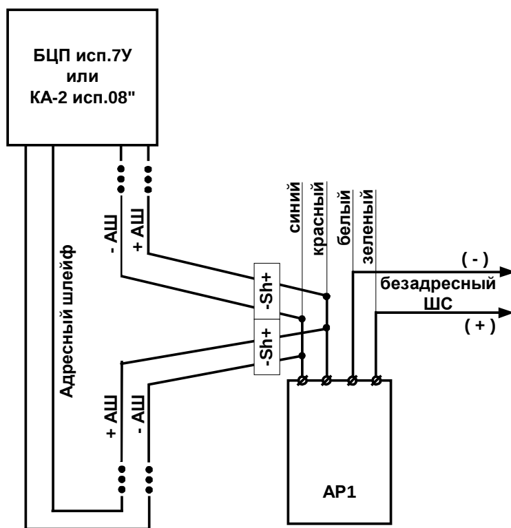
Рис. 2 Подключение СКАУ-01-Р1
