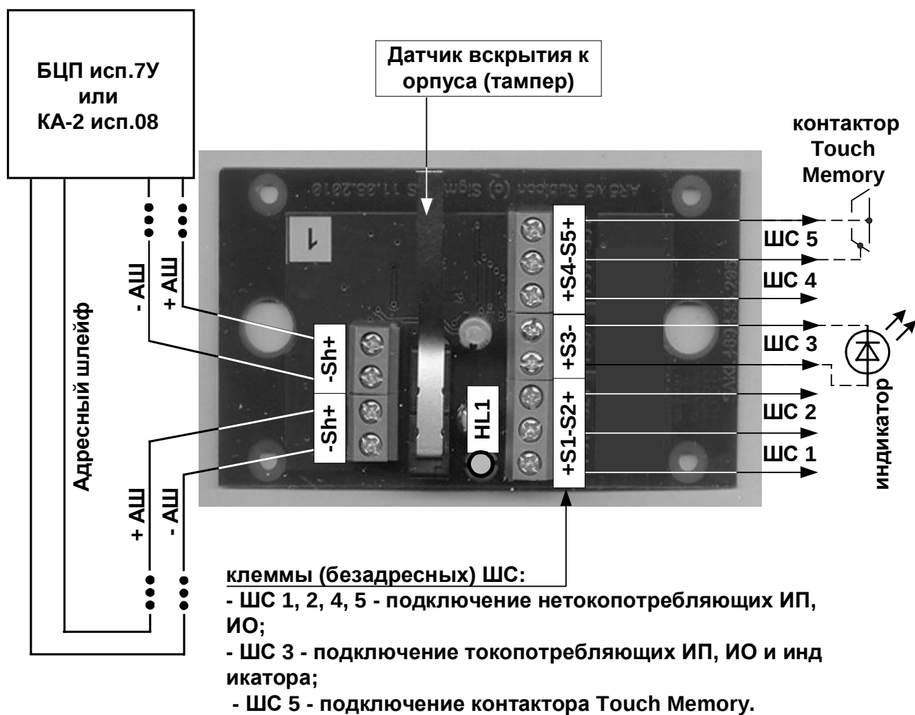
Рис. 2 Внешний вид, расположение элементов, подключение
