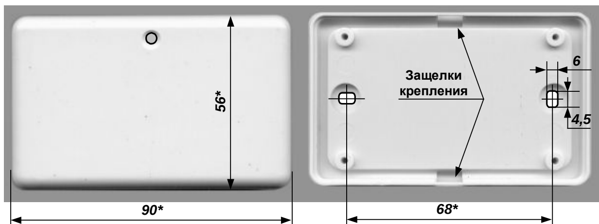
Рис. 3 Габаритные и присоединительные размеры корпуса СКАУ-01-Р5
