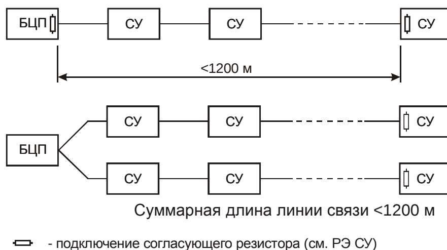
Рис. 5 Варианты включения СУ в линию связи
