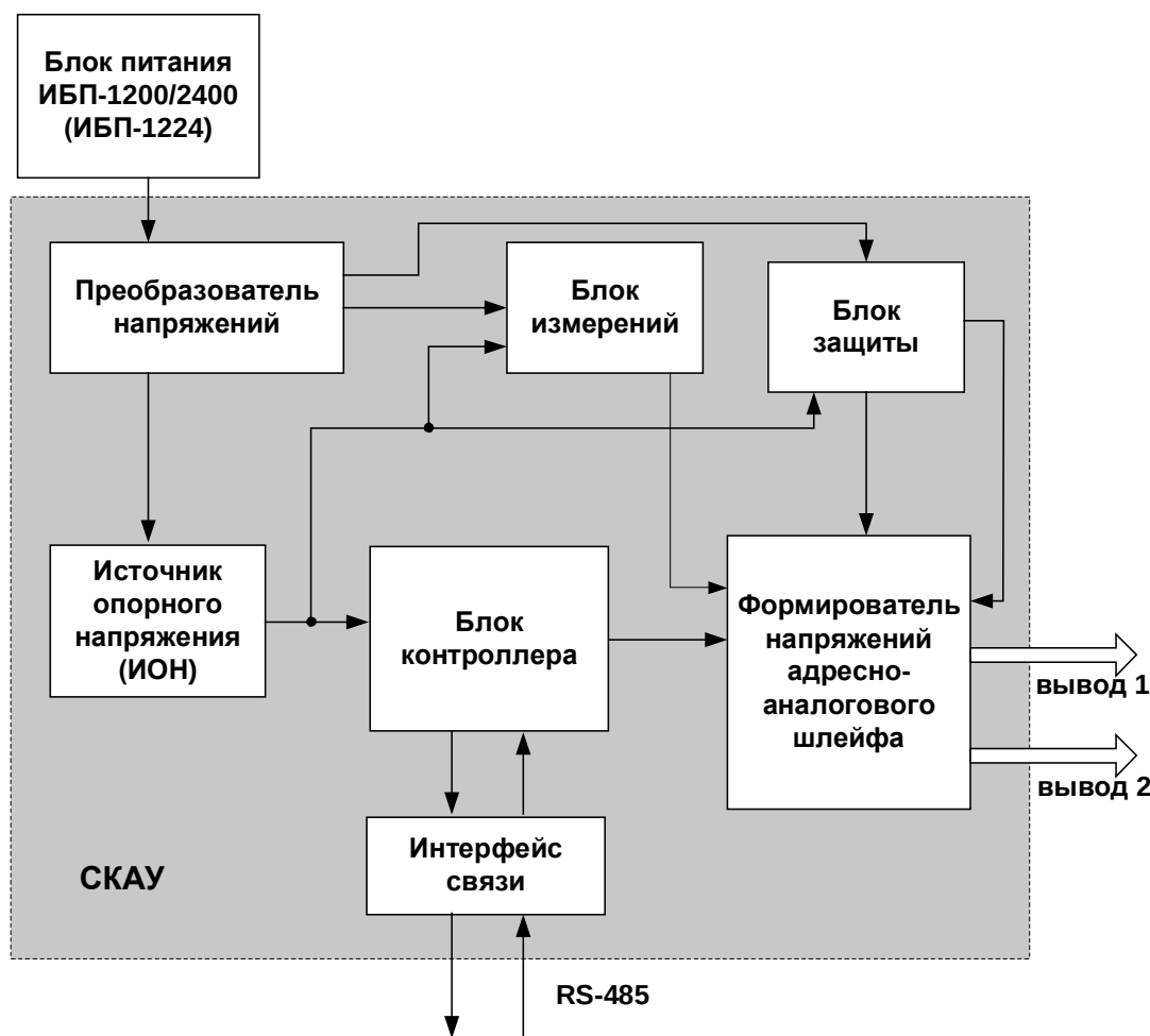
Рис. 1 Функциональная блок-схема СКАУ
