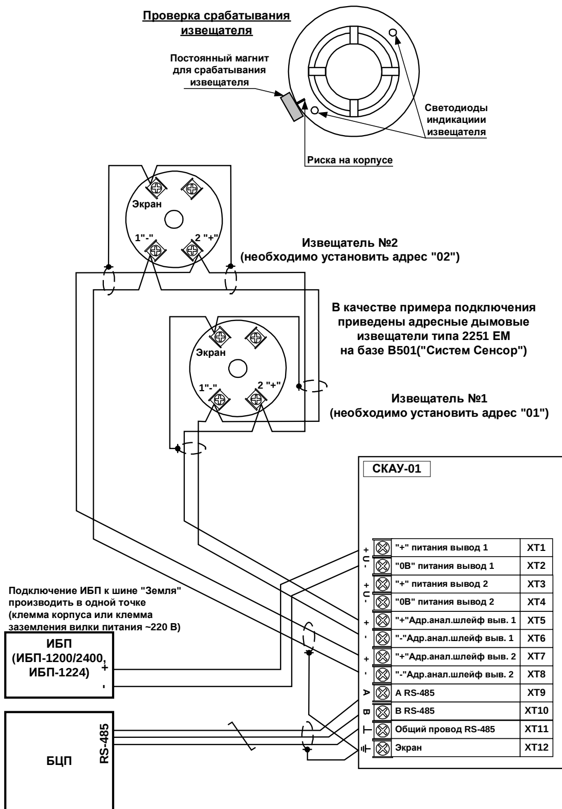
Рис. 6 Схема проверки СКАУ
