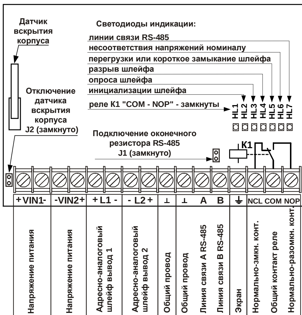
Рис. 4 Внешний вид платы
