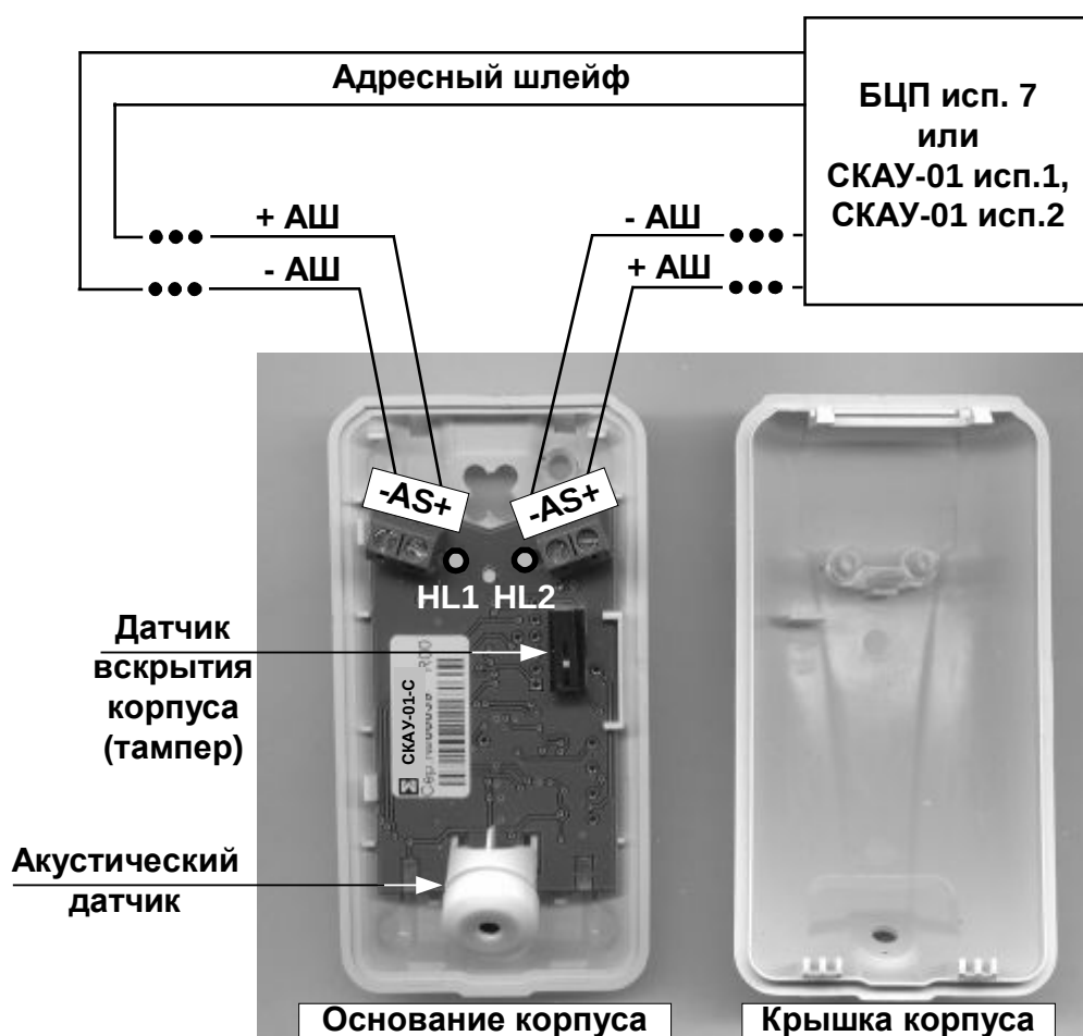
Рис. 3 Конструкция и подключение устройства
