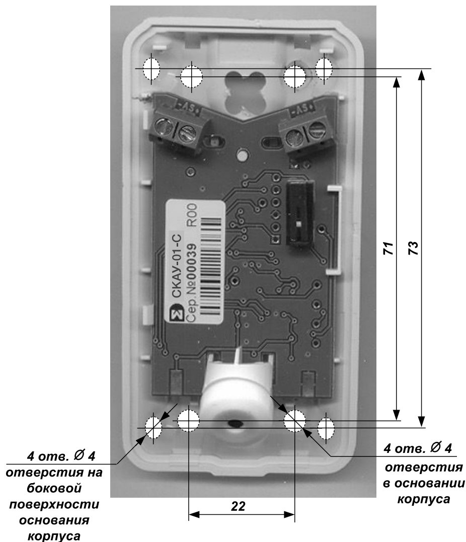
Рис. 4 Присоединительные размеры
