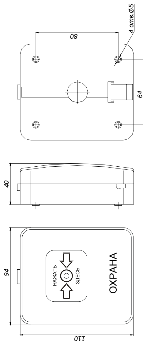
Рис. 3. СКАУ-01-Т. Габаритные и присоединительные размеры
