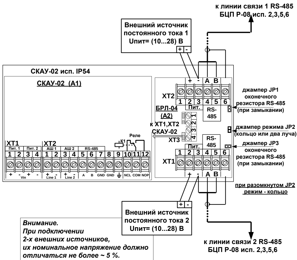
Рис. 2 Применение (подключение) СКАУ-02 IP54 в режиме кольца линий связи RS-485
