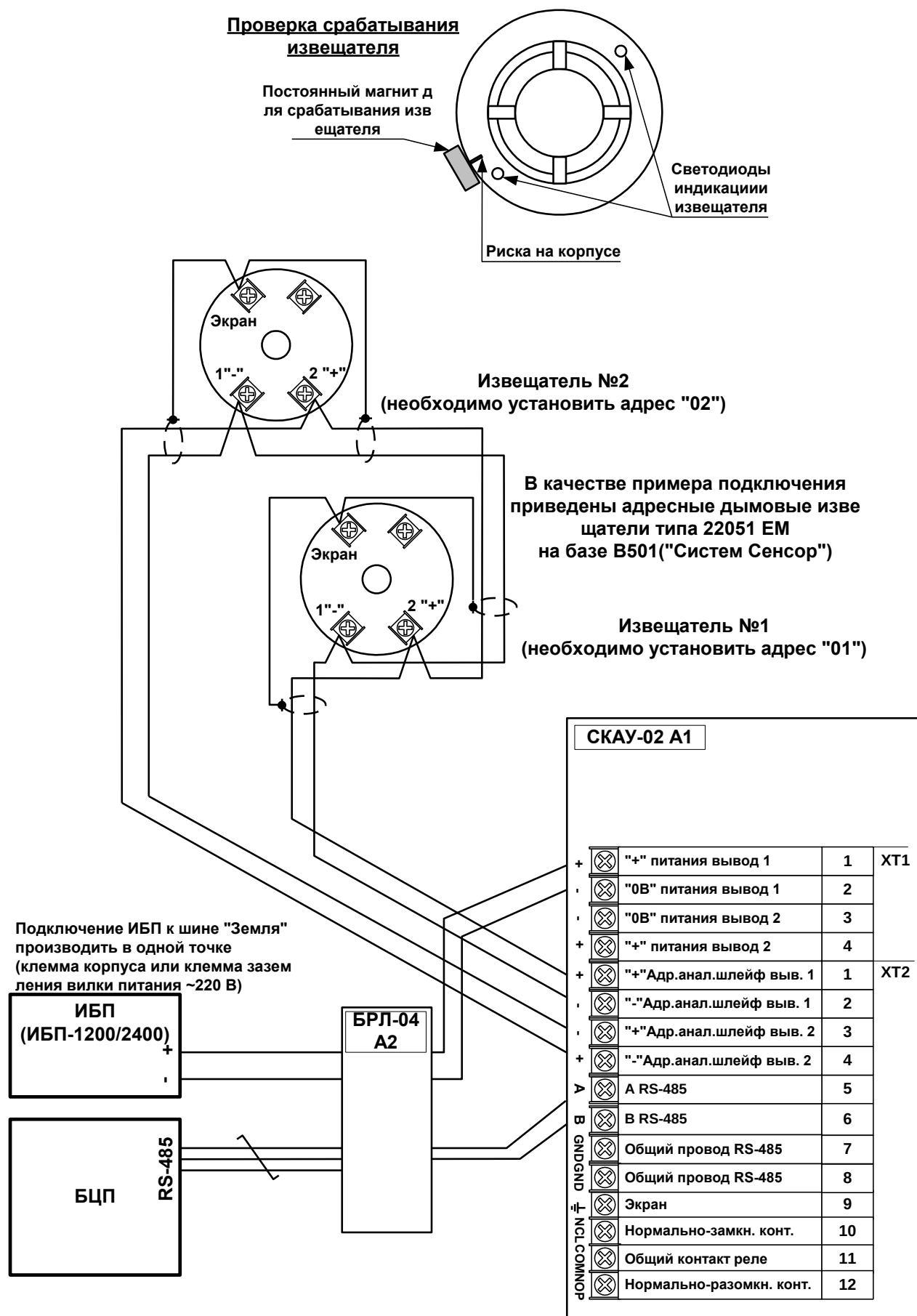
Рис. 6 Схема проверки адресного шлейфа СКАУ
