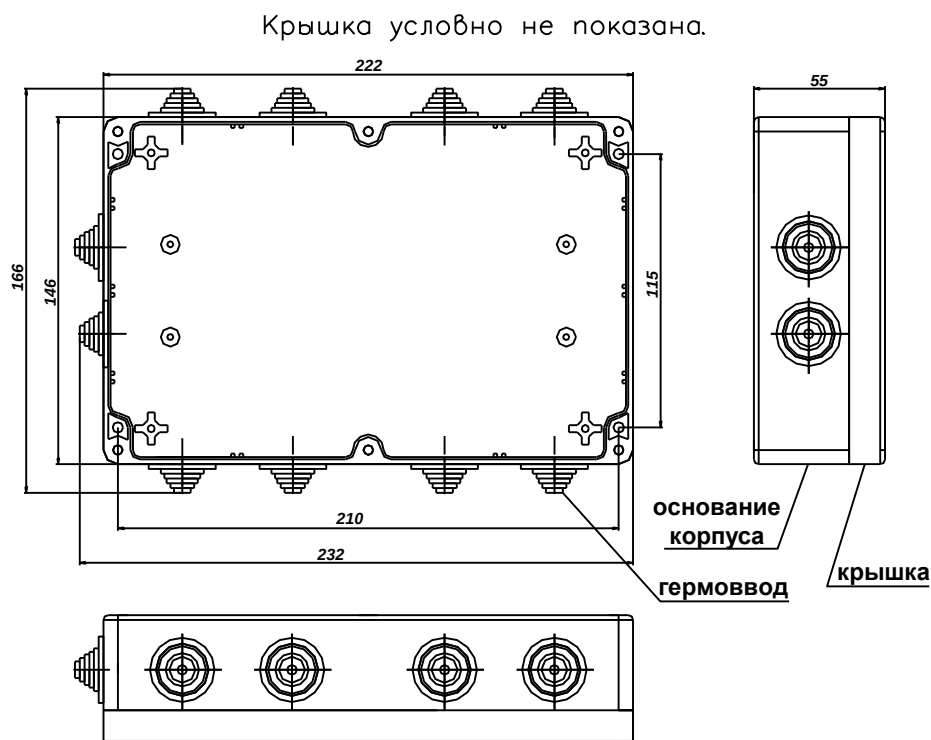
Рис. 3 Внешний вид, габаритные и присоединительные размеры
