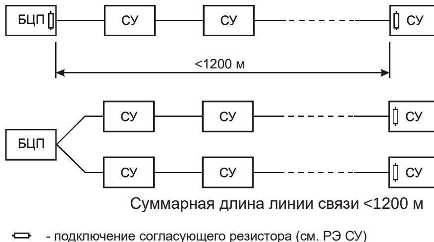
Рис. 5 Варианты включения СУ в линию связи (на нижнем рис. показано два луча)
