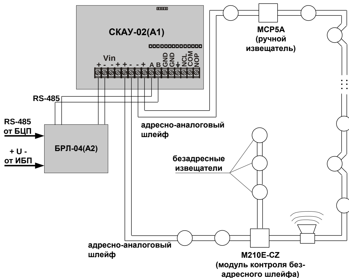
Рис. 7 Типовая схема адресных извещателей СКАУ
