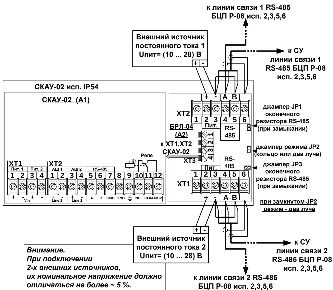
Рис. 1 Применение (подключение) СКАУ-02 IP54 в режиме двух параллельных линиях связи RS-485 (два луча)
