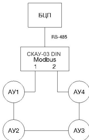
Подключение интерфейсов СКАУ-03 DIN
