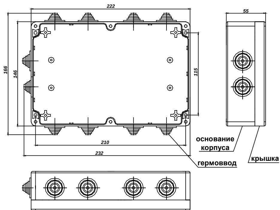
Рис. 3 Габаритные и присоединительные размеры СКИУ-01 П
