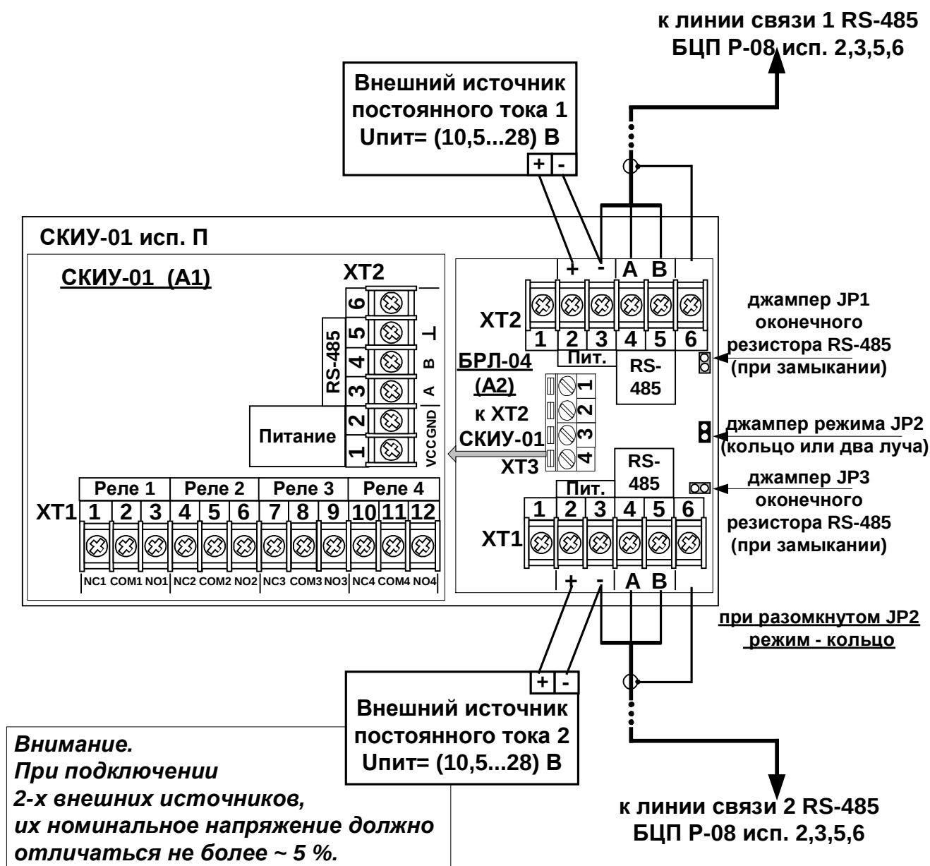
Рис. 2 Применение (подключение) СКИУ-01 П в режиме кольца линий связи RS-485
