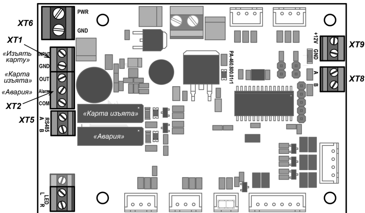
Рисунок 2. Внешний вид платы управления картоприемника
